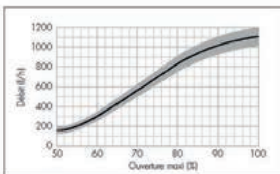
Débit vs. ouverture max. moteur - primaire ECS
