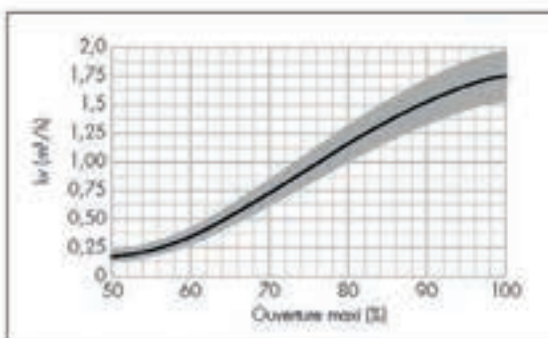
Kv vs. ouverture max. moteur - primaire chauffage
