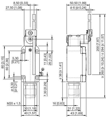
Levier à tige 8074/2--DD-40
