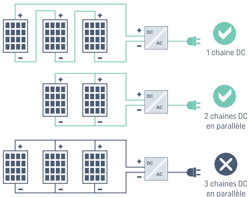
FIG. 7 : Schéma électrique simple qui montre la différence entre 1 seule et plusieurs chaînes PV
