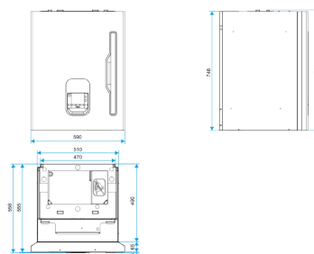
Unité supérieure T.One® AquaAIR avec façade
