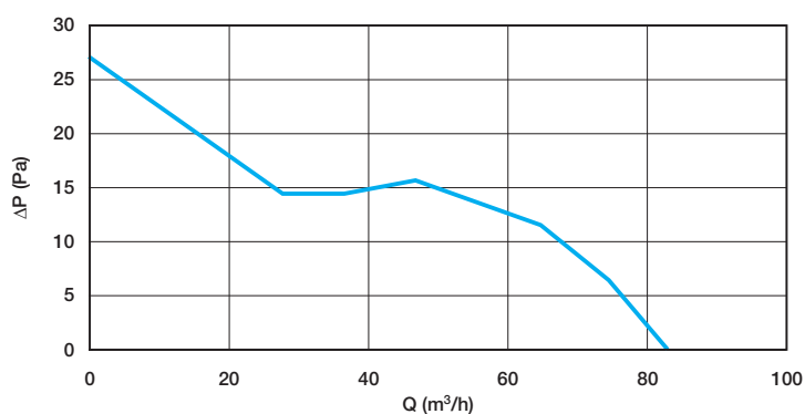
Courbe aérodynamique GRAPHIC 100
