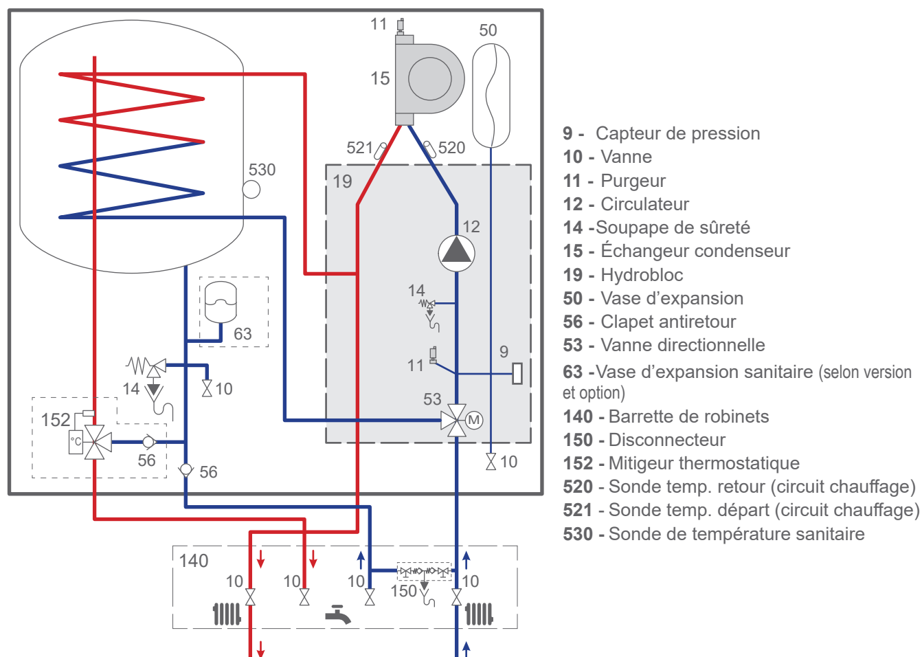
fig. 4 - Principe hydraulique
