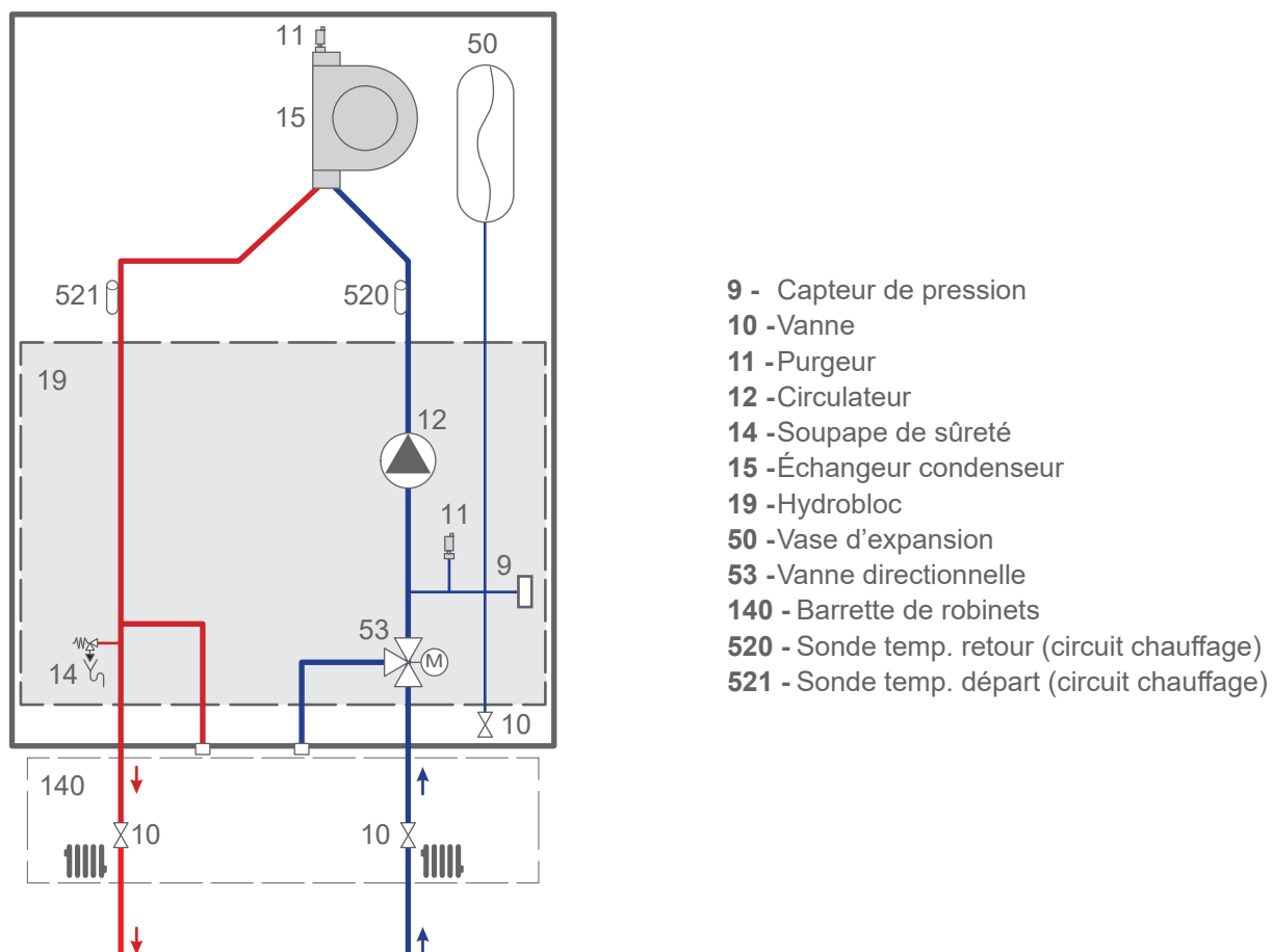
fig. 4 - Principe hydraulique
