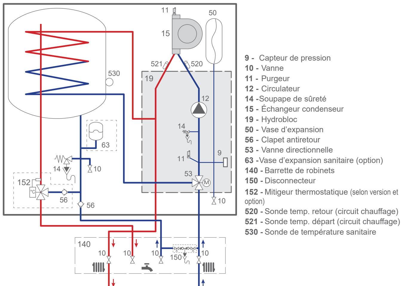
fig. 4 - Principe hydraulique
