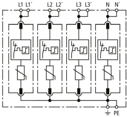
Schéma de principe du circuit DG MP TNS 275
