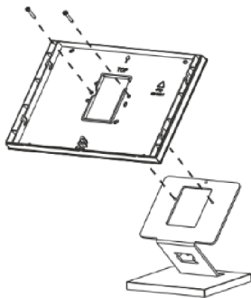
Abb. 11: Tischständer 83506-500
