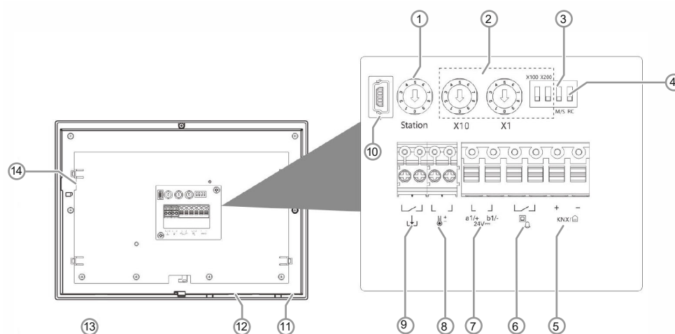
Abb. 3: Geräteübersicht ABB SmartTouch® Rückseite
