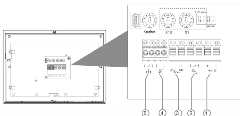
Abb. 5: Elektrischer Anschluss
