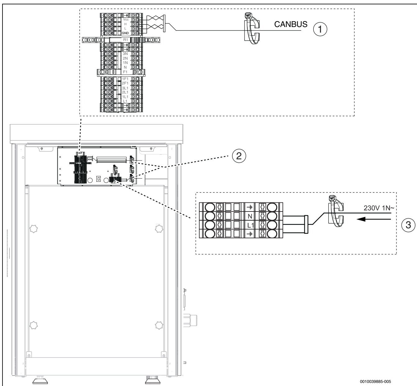
Fig. 35 Boîtier électrique
