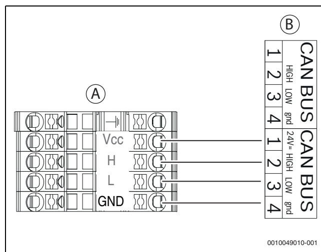
Fig. 32 CAN-BUS pompe à chaleur - unité intérieure
