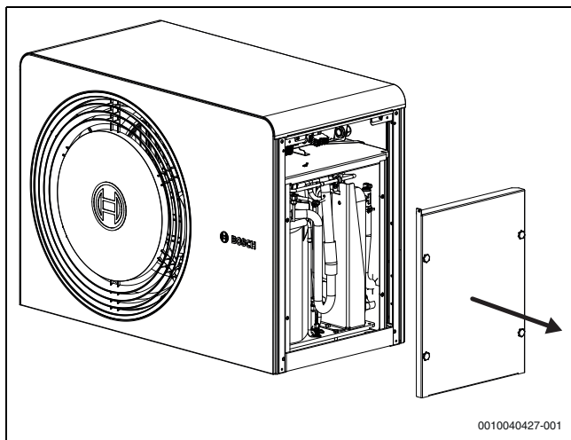
Fig. 30 Cache du boîtier du réfrigérant
