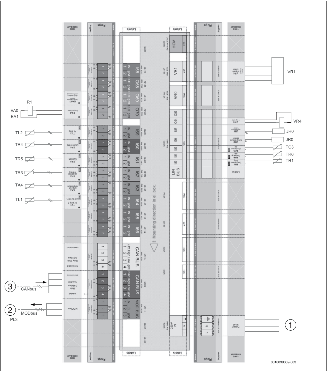
Fig. 46 Schéma de connexion XCU-SRH (XCU-HP)
