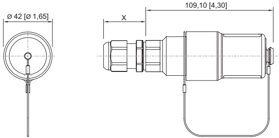
8595/1 Accouplement X = en fonction du presse-étoupe utilisé
