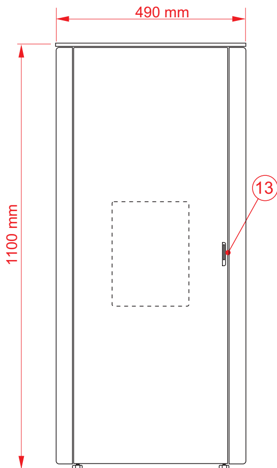
Vista frontale
