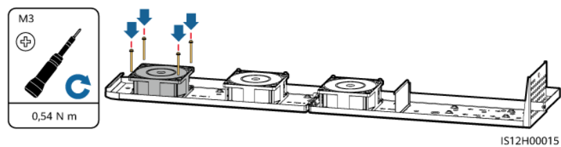
Figure 8-9 Installation d'un ventilateur
