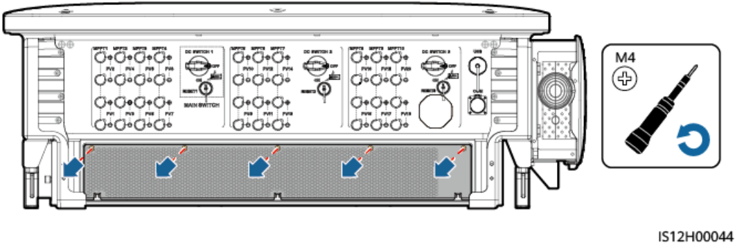
Figure 8-1 Retrait de la plaque de déflecteur de la grille d'aération d'entrée
