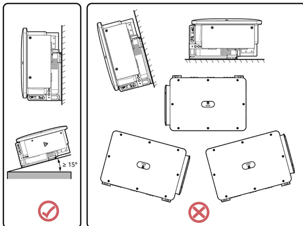
Figure 4-2 Angle d'installation
