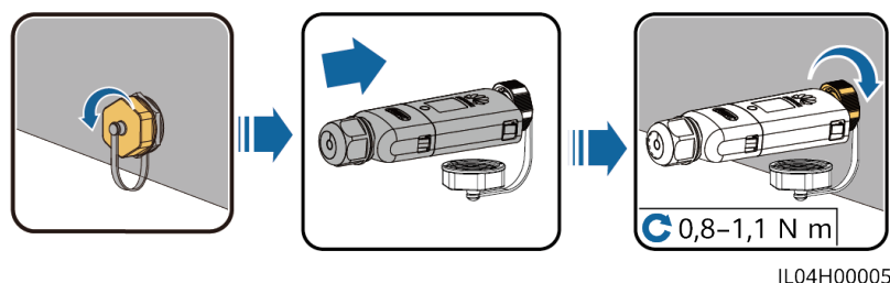
Figure 5-36 Installation du Smart Dongle WLAN-FE (SDongleA-05 pour le scénario de communication WLAN)
