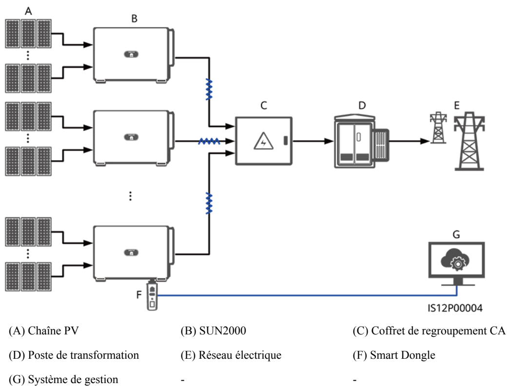
Figure 5-4 Mise en réseau du MBUS (Smart Dongle)
