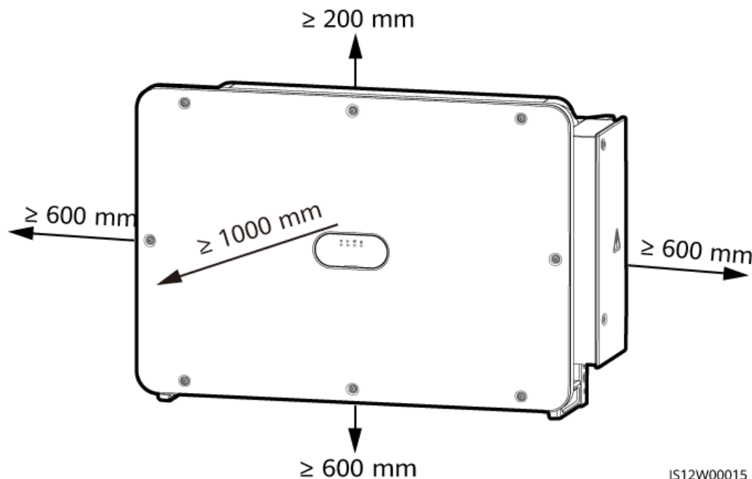
Figure 4-3 Dégagement
