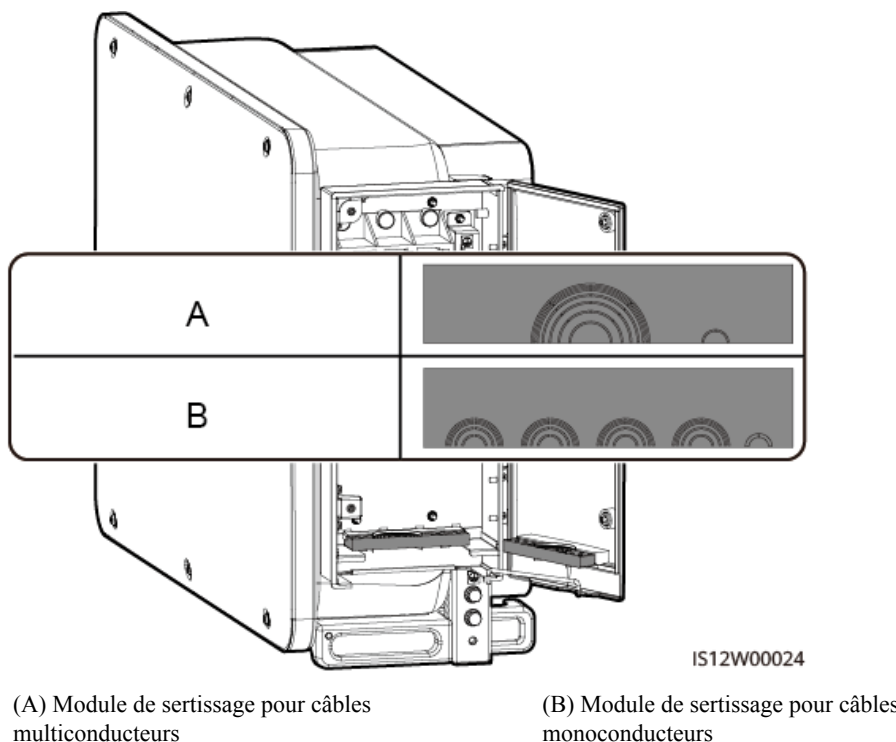
Figure 5-9 Sélection d'un module de sertissage
