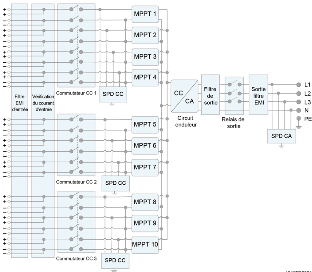
Figure 2-10 Diagramme schématique
