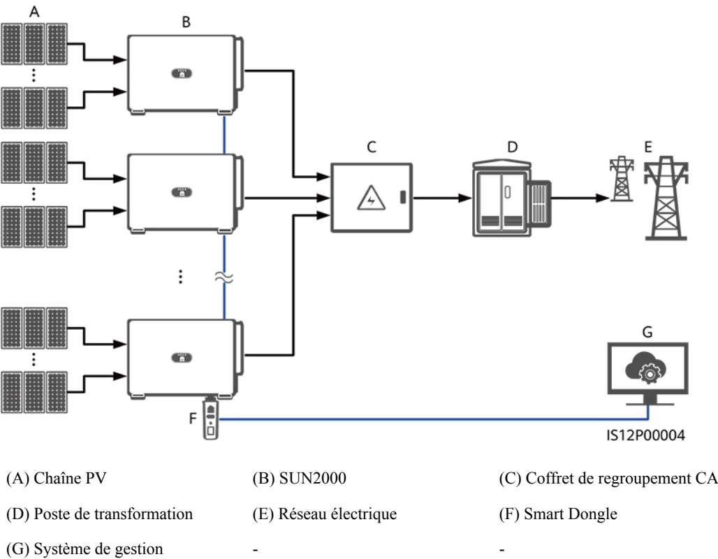
Figure 5-2 Mise en réseau RS485 (Smart Dongle)
