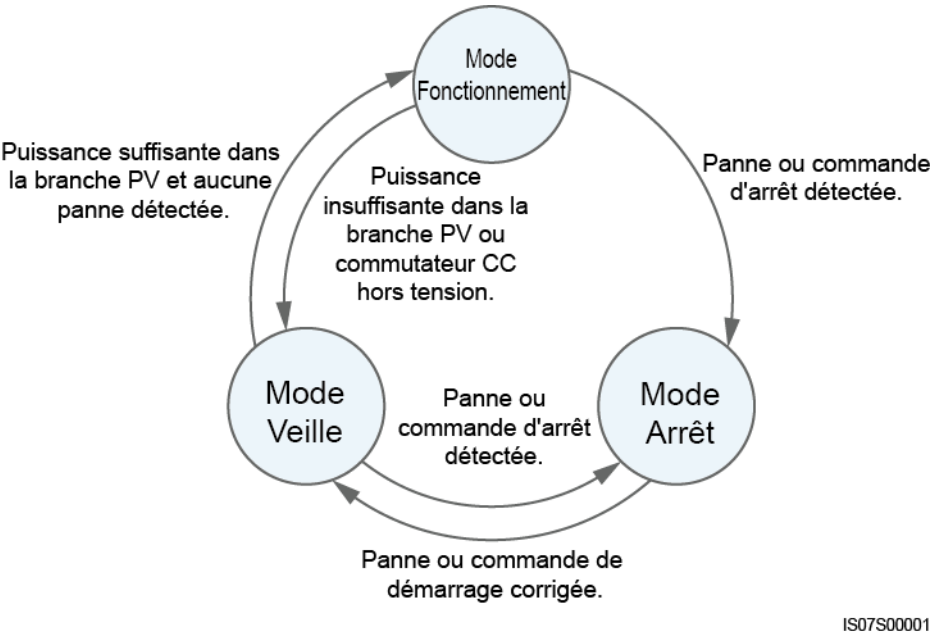
Figure 2-11 Modes de fonctionnement
