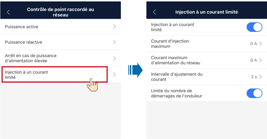
Figure 7-8 Injection à un courant limité
