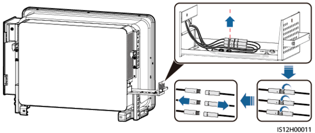
Figure 8-3 Déconnexion des câbles
