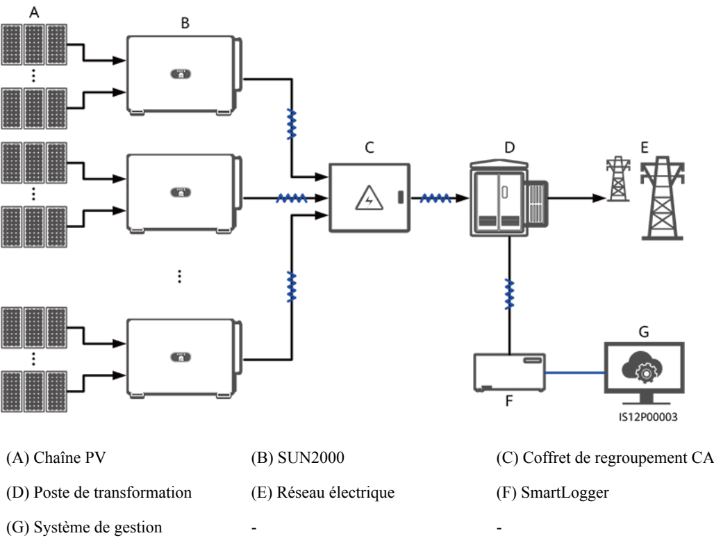
Figure 5-3 Mise en réseau du MBUS (SmartLogger)
