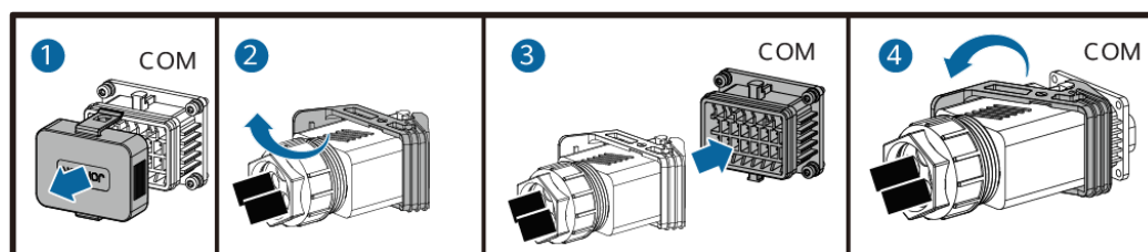
Figure 5-26 Fixation du connecteur du câble de signal
