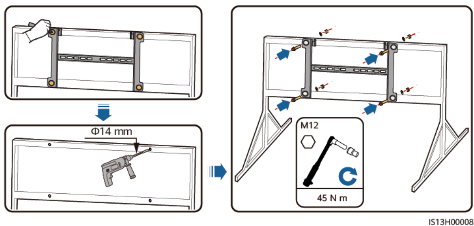
Figure 4-11 Fixation du support de montage
