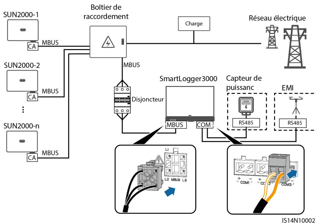
Figure 5-24 Communication MBUS (scénario C&I en Chine)
