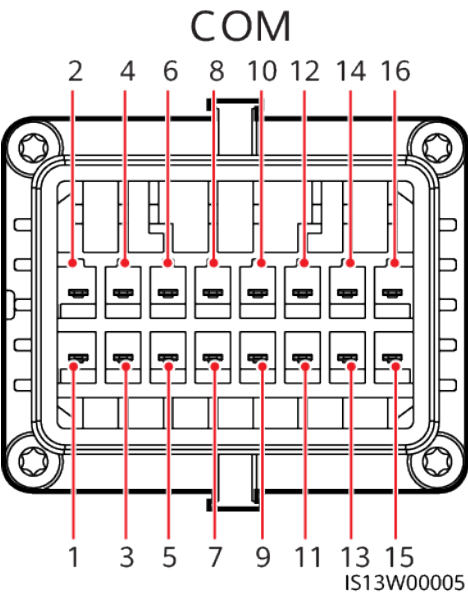
Figure 5-19 Définitions des broches
