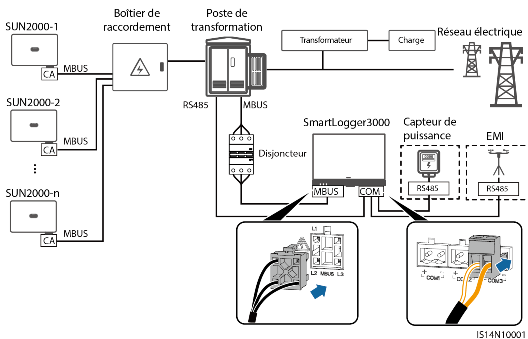
Figure 5-23 Communication MBUS (scénarios à l'échelle industrielle)
