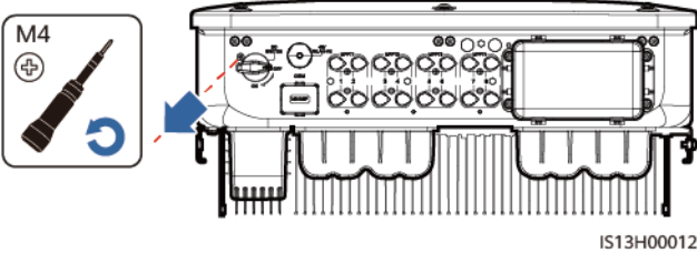
Figure 6-1 Retrait de la vis de verrouillage du DC SWITCH
