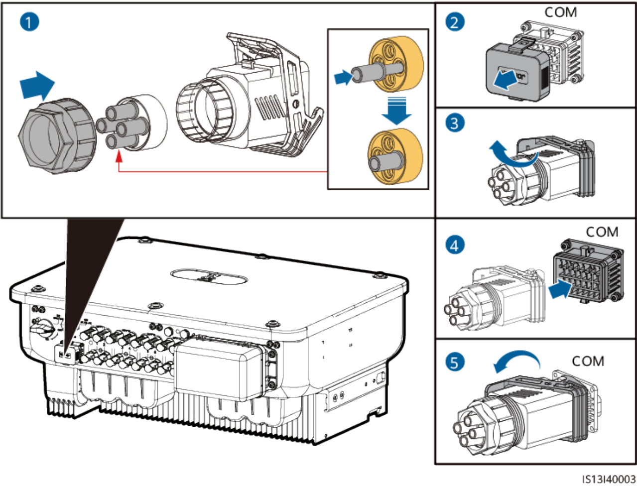
Figure 5-20 Connexion du connecteur du câble de signal
