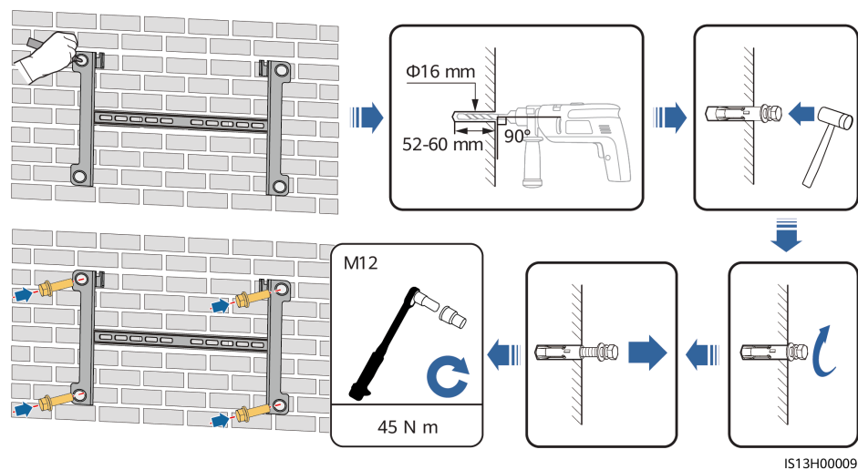
Figure 4-13 Installation d'un boulon à expansion
