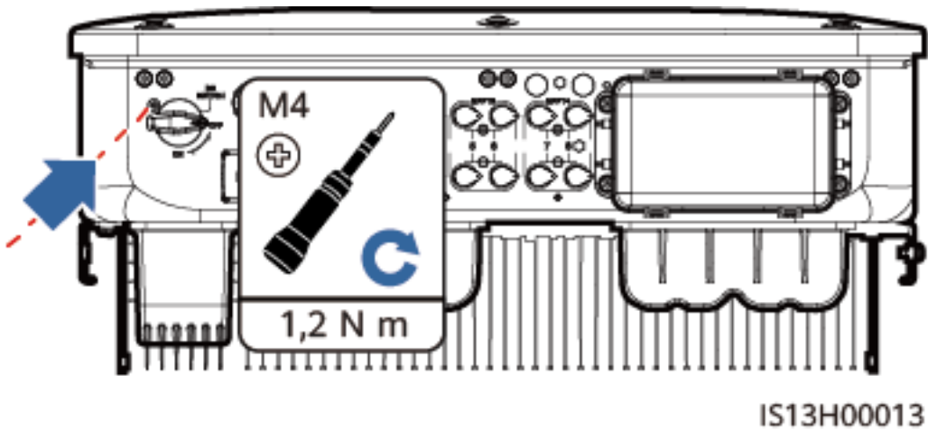
Figure 8-1 Installation de la vis de verrouillage du commutateur CC
