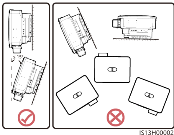
Figure 4-1 Angle d'installation
