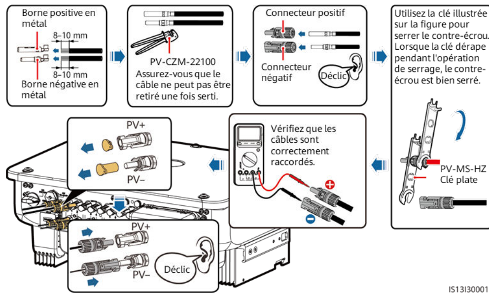
Figure 5-14 Connexion des câbles d'alimentation CC
