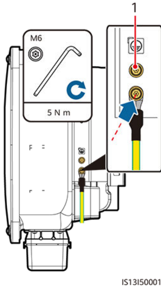
Figure 5-3 Raccordement du câble PE
