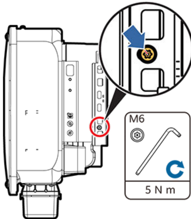
Figure 4-16 Serrage de l'écrou
