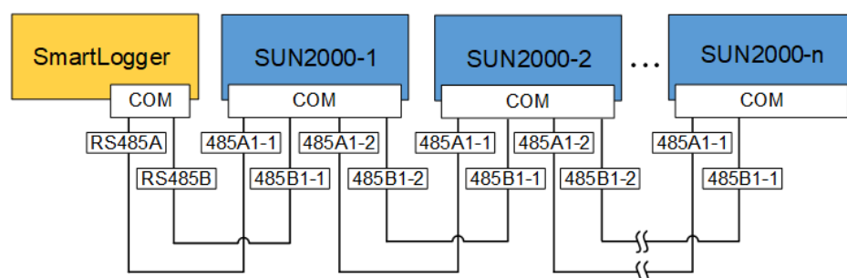
Figure 5-22 Mise en réseau du SmartLogger
