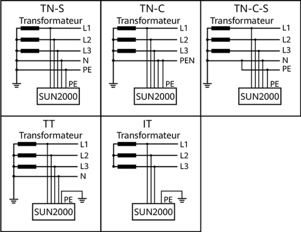
Figure 2-3 Systemes de mise à la terre
