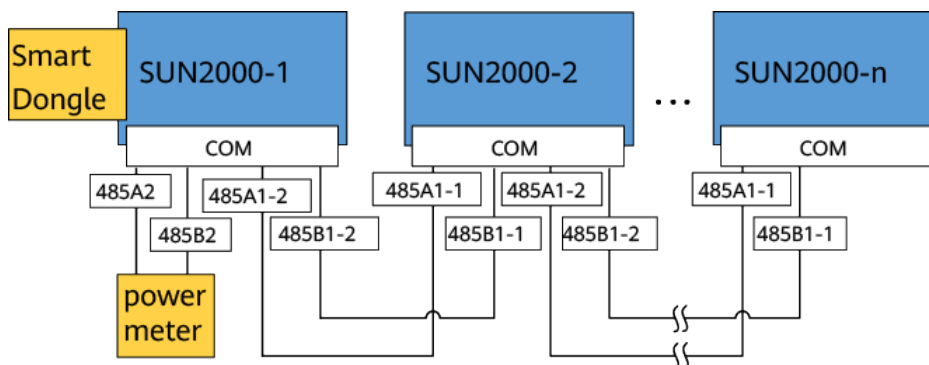
Figure 5-21 Mise en réseau du Smart Dongle
