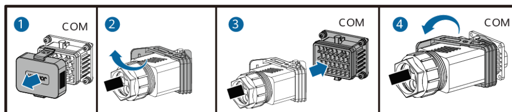
Figure 5-28 Fixation du connecteur du câble de signal
