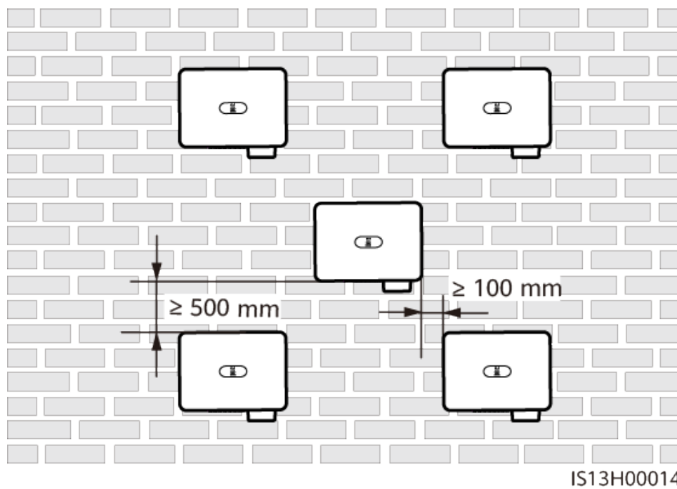
Figure 4-5 Mode d'installation en triangle à trois couches (non recommandé)
