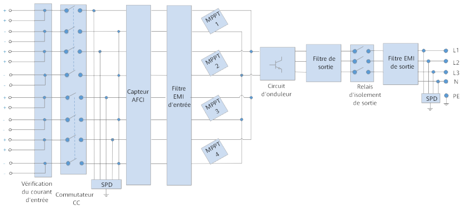
Figure 2-5 Diagramme schématique
