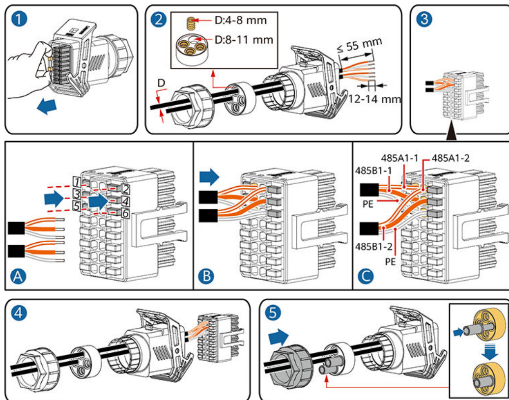
Figure 5-25 Connexion du câble
