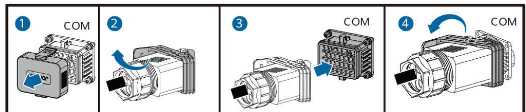
Figure 5-32 Fixation du connecteur du câble de signal
