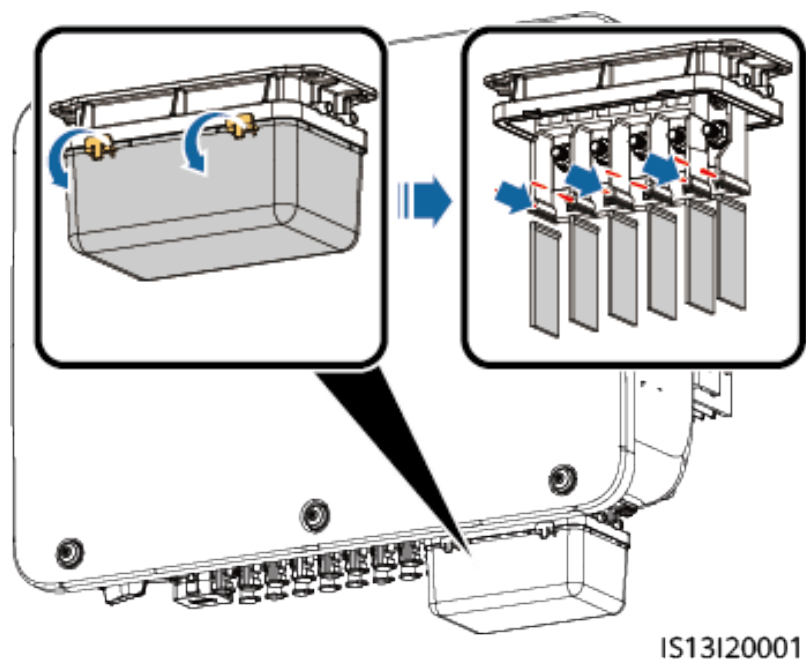
Figure 5-5 Retrait du boîtier de la borne CA
