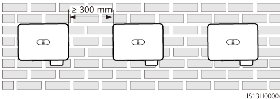
Figure 4-3 Mode d'installation horizontal (recommandé)
