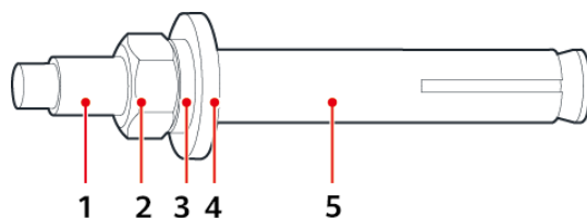
Figure 4-12 Structure d'un boulon à expansion
