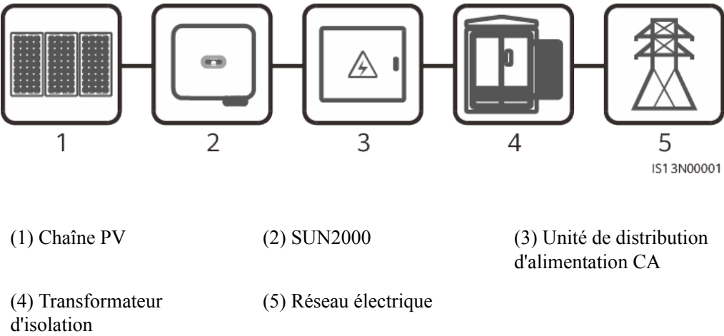
Figure 2-2 Application de mise en réseau - scénario avec un onduleur simple
