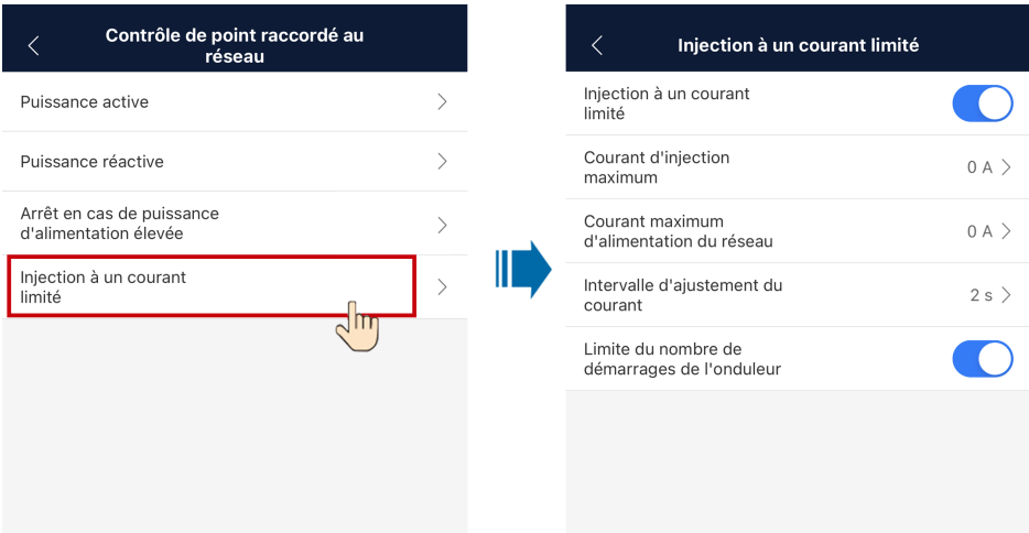
Figure 7-6 Injection à un courant limité
