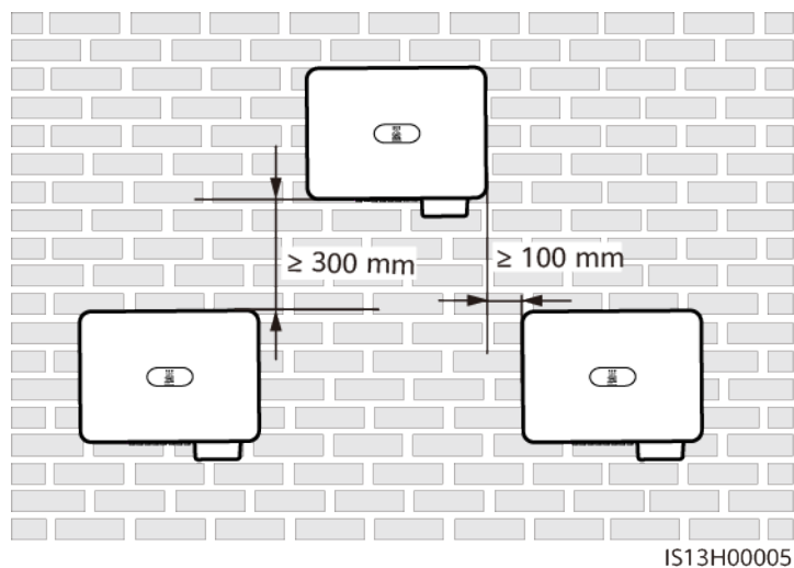
Figure 4-4 Mode d'installation en triangle (recommandé)
