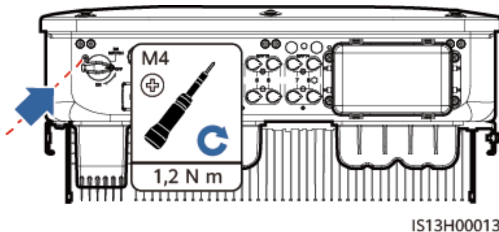
Figure 4-14 Installation de la vis de verrouillage du commutateur CC
