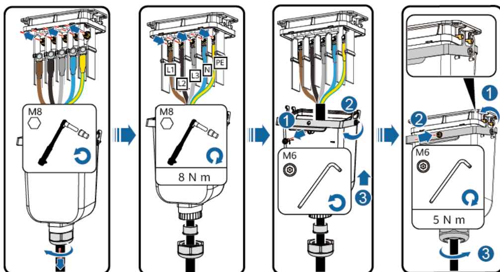
Figure 5-7 Câble à cinq conducteurs (L1, L2, L3, N et PE)
