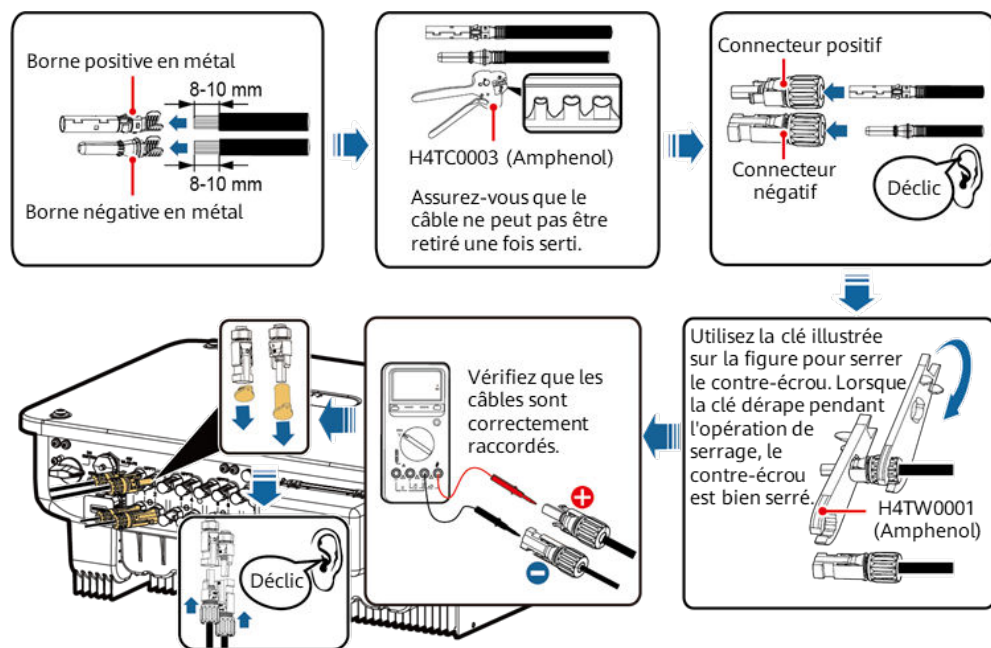
Figure 5-13 Connexion des câbles d'alimentation CC
