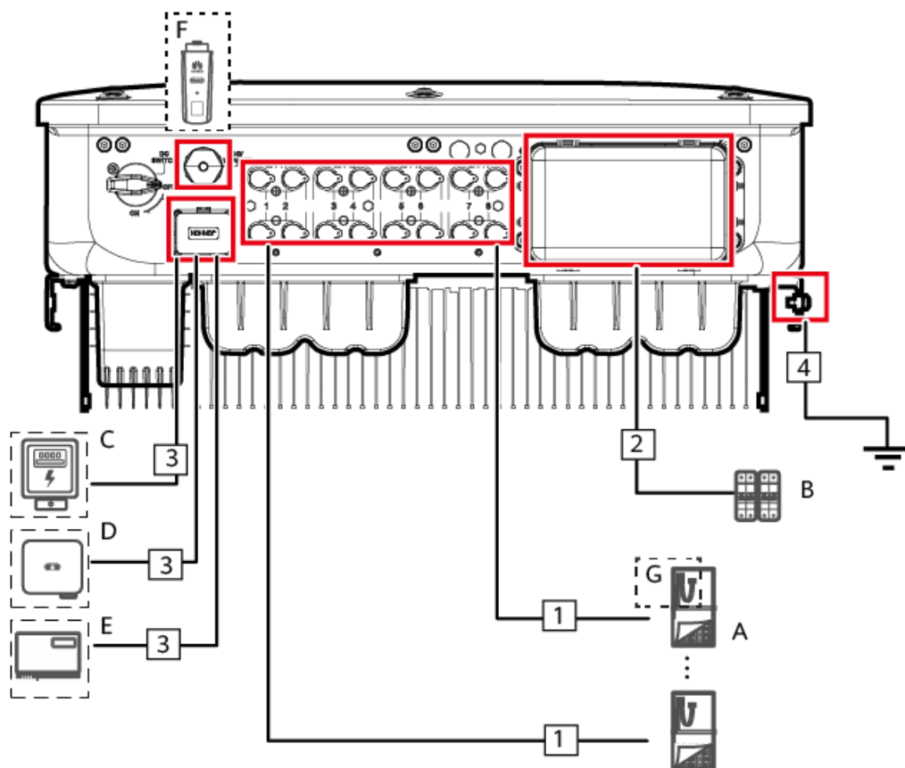
Figure 5-1 Connexions des câbles du SUN2000 (les composants dans l'encadré en pointillé sont facultatifs)
