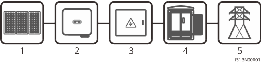
Figure 2-2 Application de mise en réseau – scénario avec un onduleur simple
