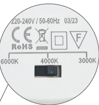
Température de couleur réglable par DIP switch
