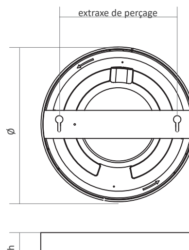
Schéma technique
