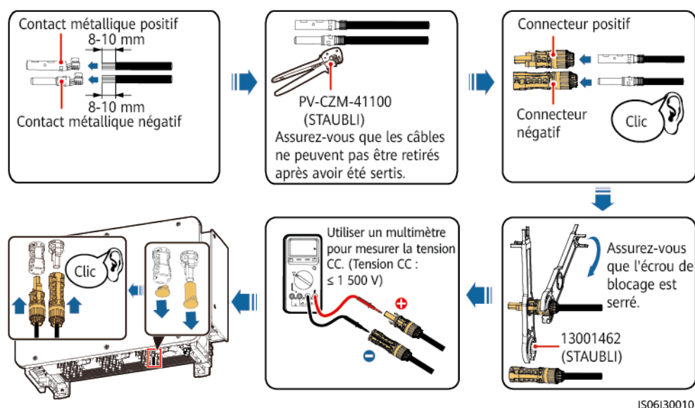
Figure 5-17 Connexion de câble
