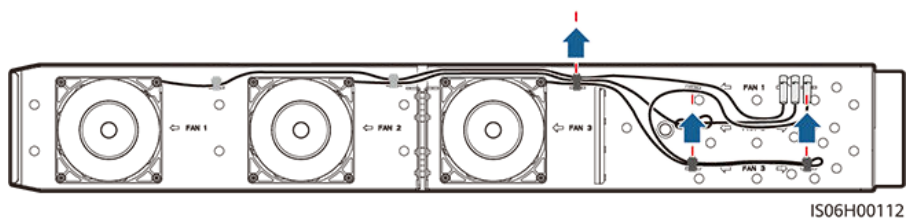
Figure 8-8 Retrait des serre-câbles du FAN 3
