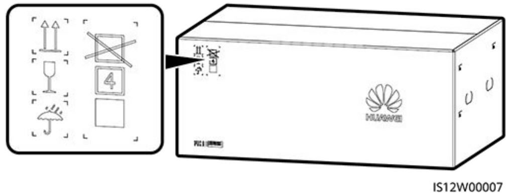
Figure 3-2 Nombre maximal de couches d'empilage
