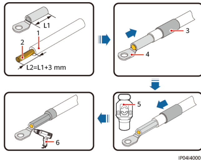
Figure 5-4 Sertissage d'une borne DT
