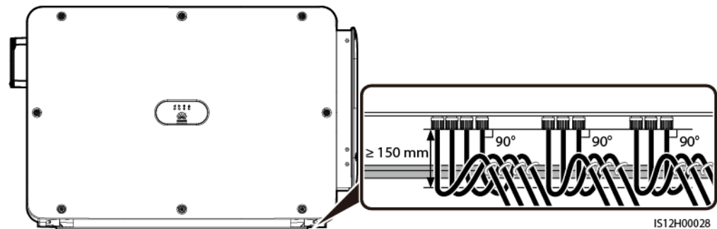
Figure A-6 Liaison des connecteurs en Y
