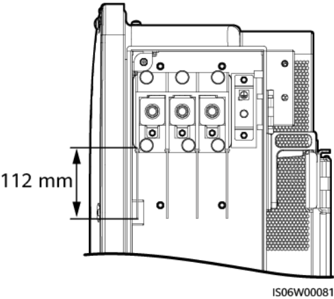
Figure 5-10 Spécifications du déflecteur en caoutchouc
