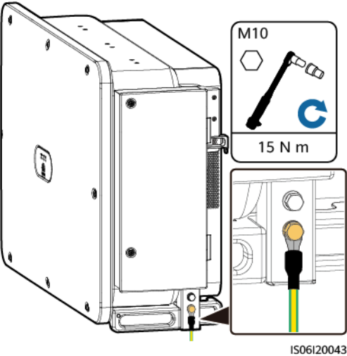
Figure 5-11 Connexion de câble
