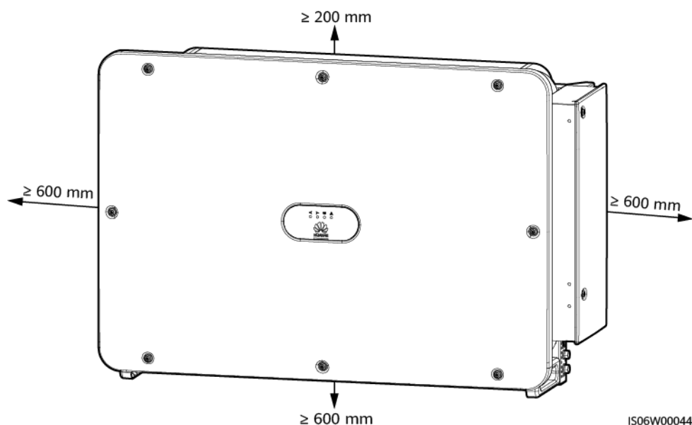
Figure 4-2 Espace d'installation
