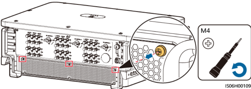
Figure 8-2 Retrait du déflecteur
