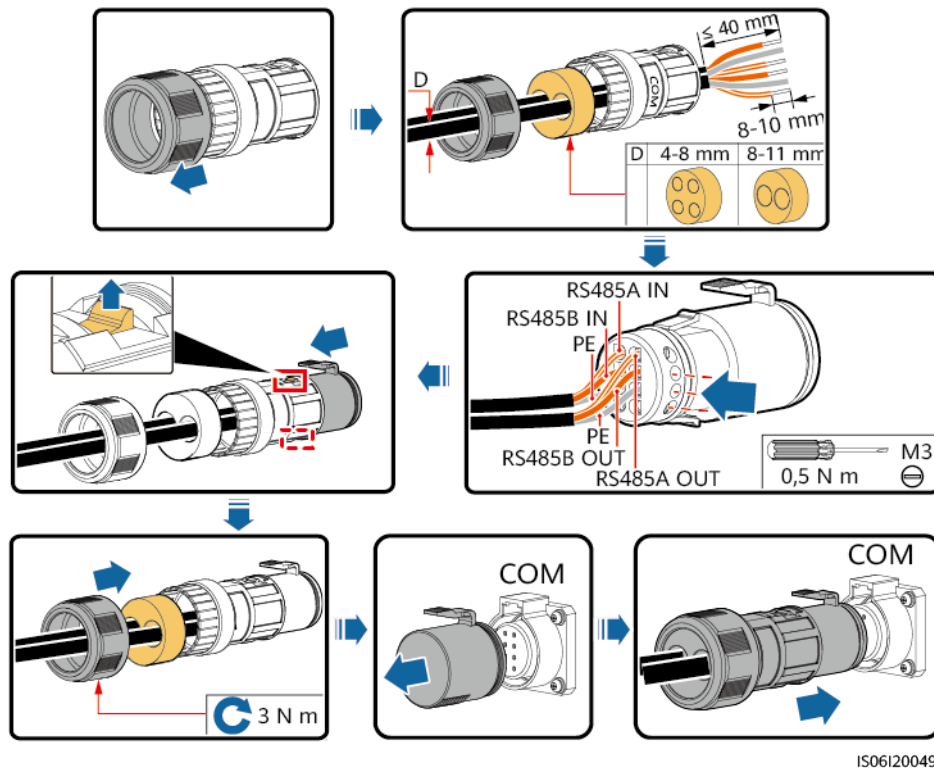
Figure 5-21 Raccordement de câble (fiche en caoutchouc à quatre trous 4–8 mm)
