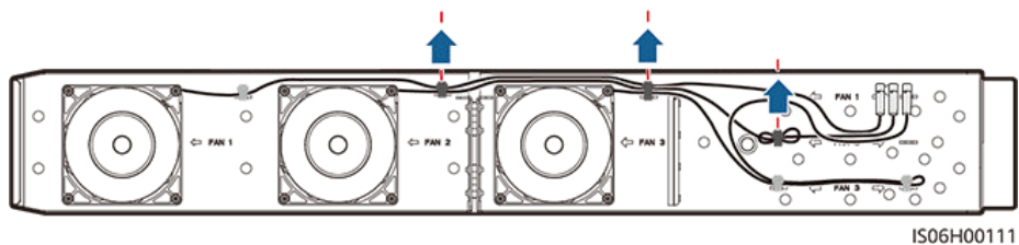
Figure 8-7 Retrait des serre-câbles du FAN 2
