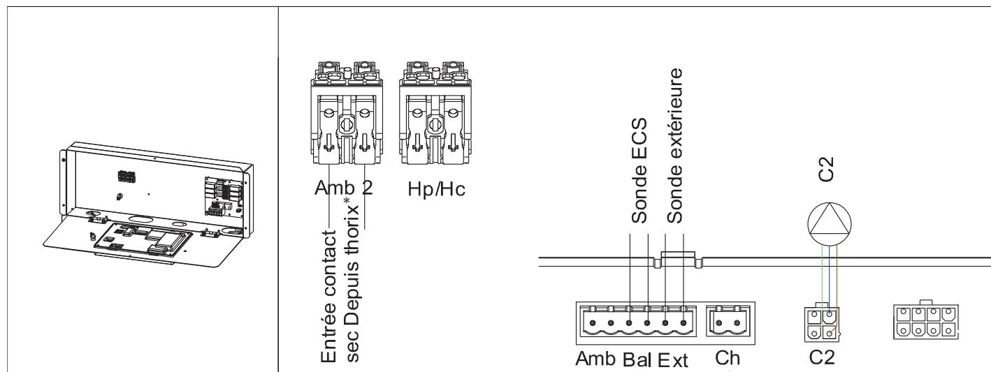
Schéma 36.23.056
