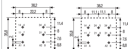
62.22 - 4300 Vue coté cuivre
