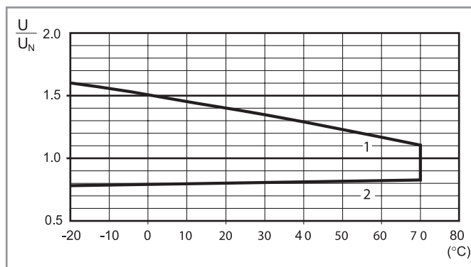
R 62 - Plage de fonctionnement bobine AC en fonction de la température ambiante - Type inverseur
