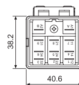
062.08 avec relais monté
