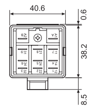
062.07 avec relais monté
