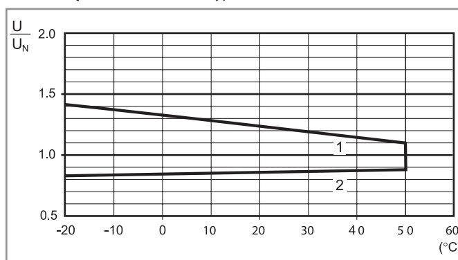
R 62 - Plage de fonctionnement bobine AC en fonction de la température ambiante - Type NO
