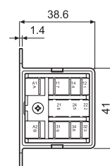
062.60 avec relais monté
