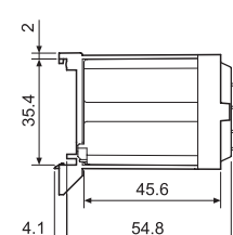
062.07 avec relais monté
