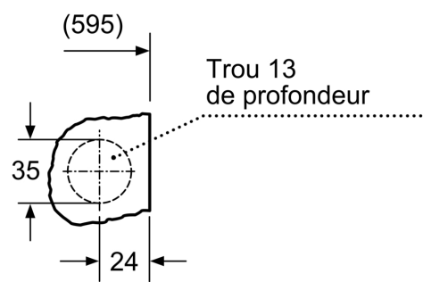
Détail Z
