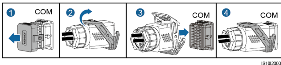
Figure 5-35 Fixation du connecteur du câble de signal
