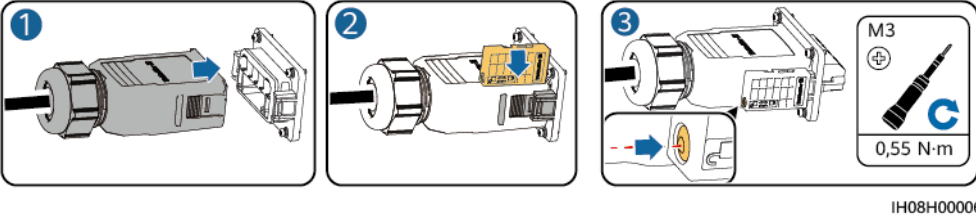
Figure 5-9 Fixation du connecteur CA
