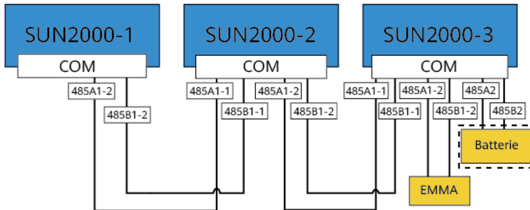
Figure 5-19 Mise en réseau EMMA (les composants dans les encadrés en pointillé sont facultatifs)
