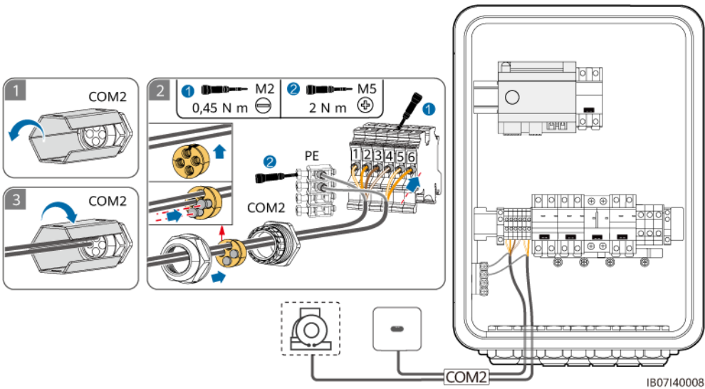
Figure 5-19 Connexion du câble de signal du SmartGuard (la case en pointillée indique un composant facultatif)
