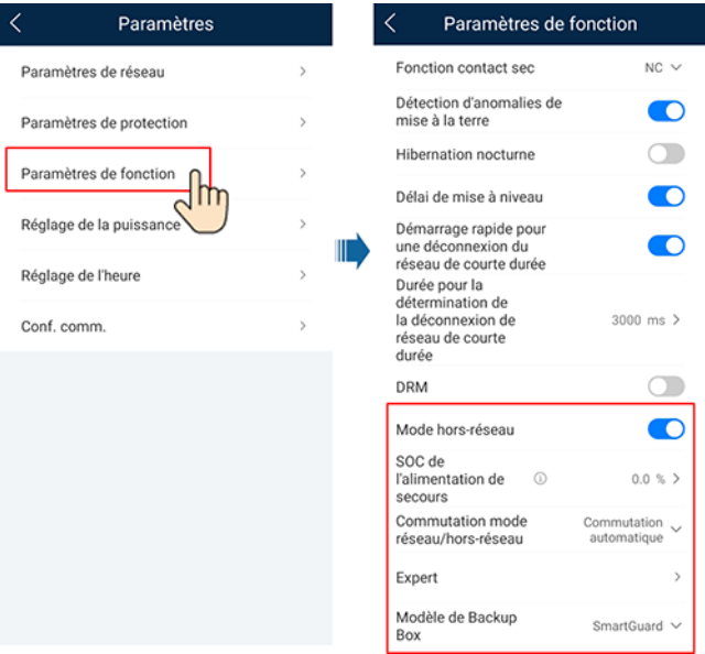
Figure 6-6 Réglage du mode hors-réseau
