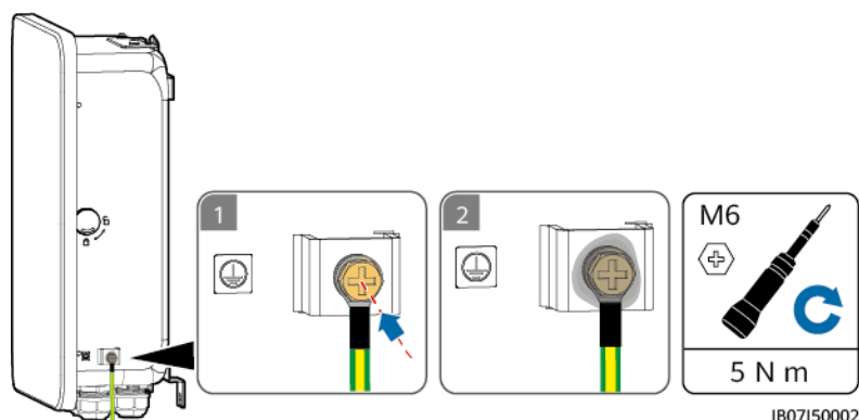
Figure 5-4 Connexion du câble PE
