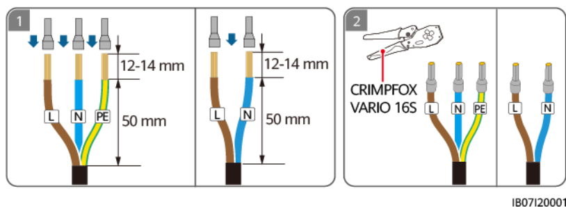
Figure 5-16 Sertissage des bornes d'extrémité du cordon CA
