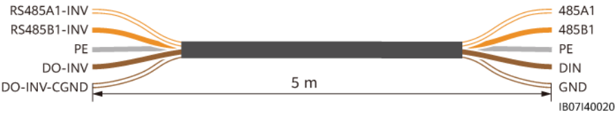
Figure 5-2 Câble de signal (acheté auprès de Huawei) connectant le SmartGuard à l'onduleur
