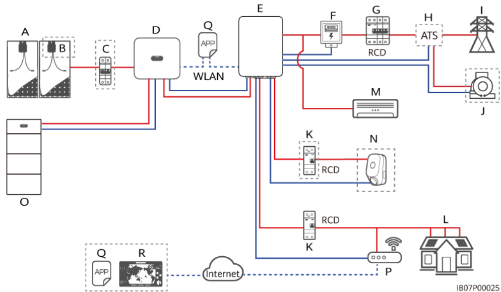
Figure 2-5 Mise en réseau avec certaines charges connectées au SmartGuard (composants optionnels indiqués par des cadres en pointillés)
