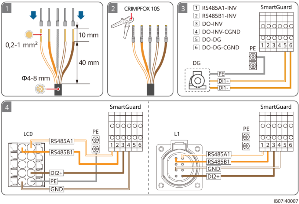
Figure 5-18 Sertissage des bornes d'extrémité du cordon pour le câble de signal (la case en pointillée indique un composant facultatif)
