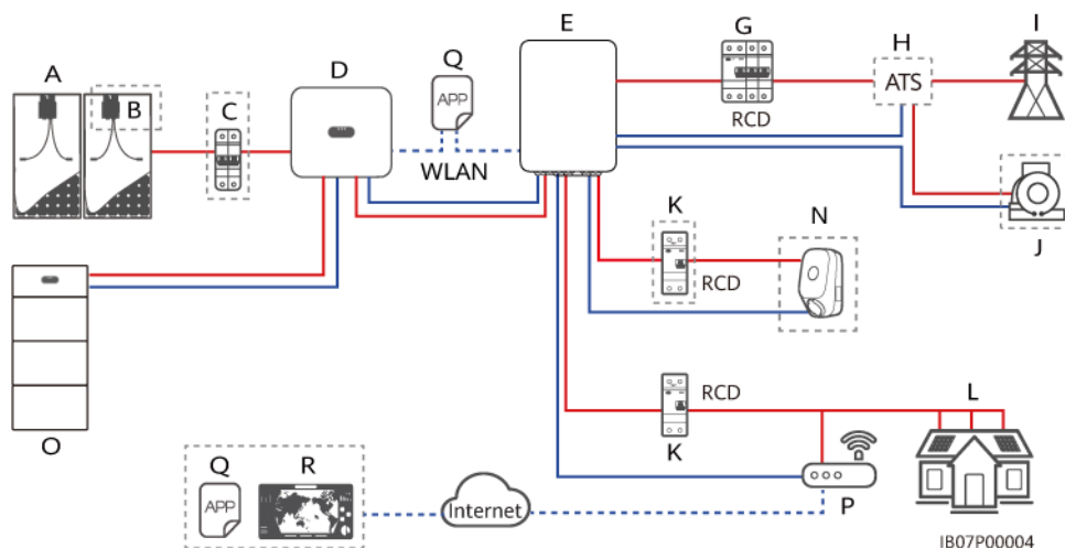
Figure 2-4 Mise en réseau avec toutes les charges connectées au SmartGuard (composants optionnels indiqués par des cadres en pointillés)
