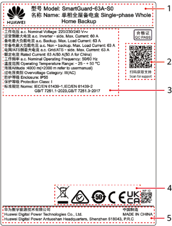
Figure 2-12 Plaque signalétique (SmartGuard-63A-S0 par exemple)
