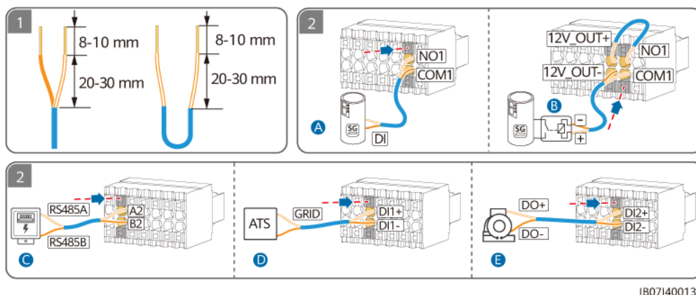
Figure 5-22 Connexion du câble de signal à la borne à 14 broches
