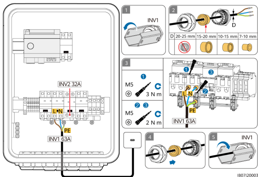
Figure 5-11 Connexion du câble d'alimentation d'entrée CA de l'onduleur
