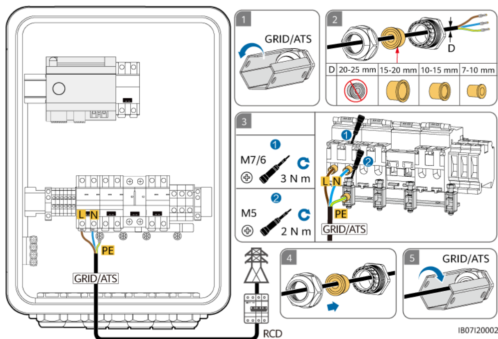
Figure 5-9 Connexion du câble d'alimentation de sortie CA du réseau
