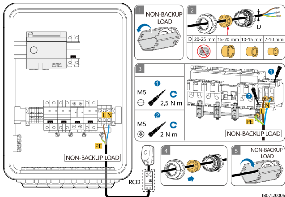
Figure 5-17 Connexion du câble d'alimentation de sortie de charge non secours (le composant dans la boîte en pointillés est optionnel)
