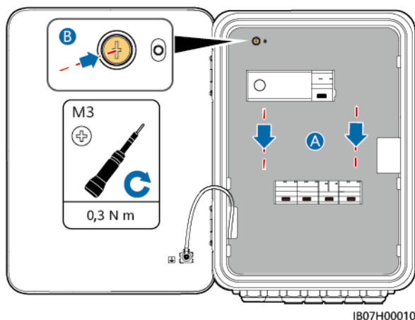
Figure 6-1 Fermeture du couvercle
