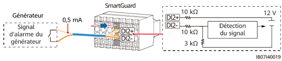
Figure E-2 Signal d'alarme du générateur
