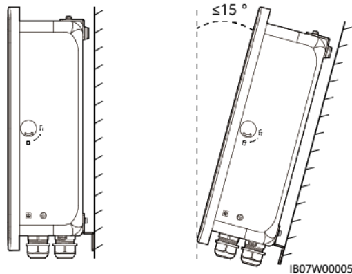
Figure 4-3 Angle d'installation
