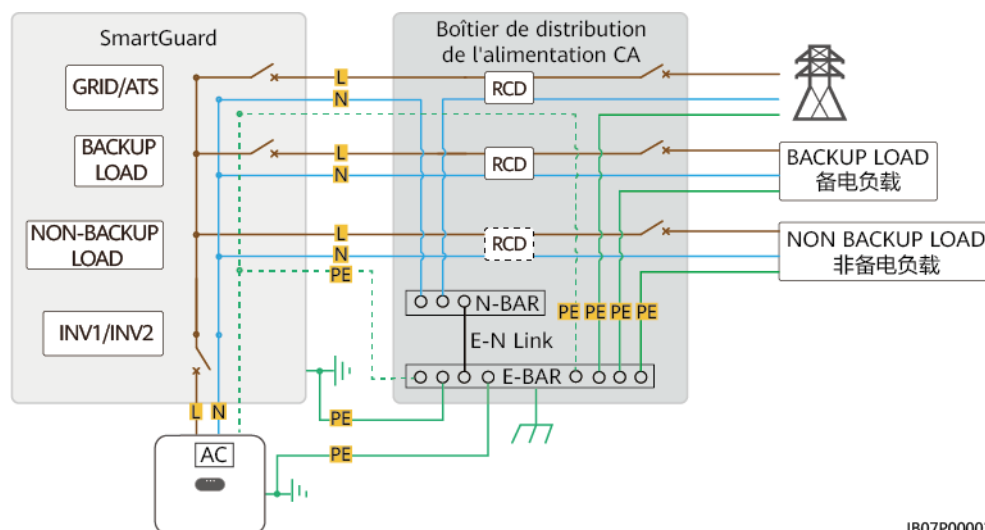
Figure 2-3 Schéma de câblage résidentiel du SmartGuard-63A-AUS0 (les lignes pointillées indiquent les connexions de câble optionnelles)
