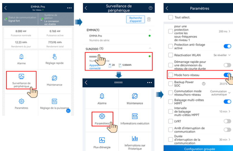
Figure 6-5 Réglage du mode hors-réseau
