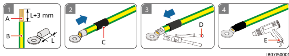
Figure 5-3 Sertissage d'une borne OT
