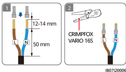
Figure 5-13 Sertissage des bornes d'extrémité du cordon CA SmartGuard-63A-AUS0
