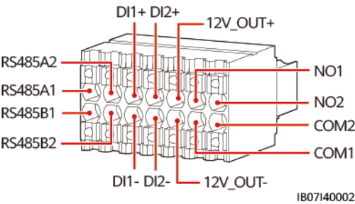
Figure 5-21 Définitions des broches
