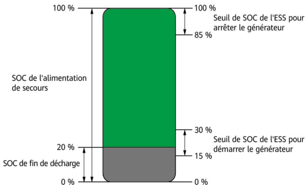
Figure 6-10 SOC Batterie
