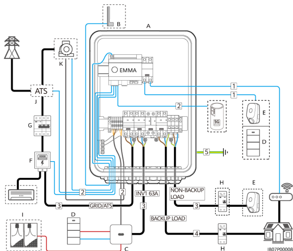
Figure 5-1 Connexions des câbles (configuration optionnelle indiquée par des cadres en pointillés)
