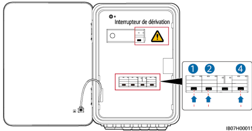
Figure 6-2 Mise sous tension les interrupteurs
