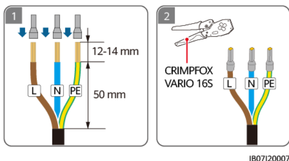
Figure 5-12 Sertissage des bornes d'extrémité du cordon CA SmartGuard-63A-S0
