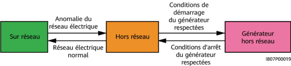
Figure 2-11 Modes de fonctionnement
