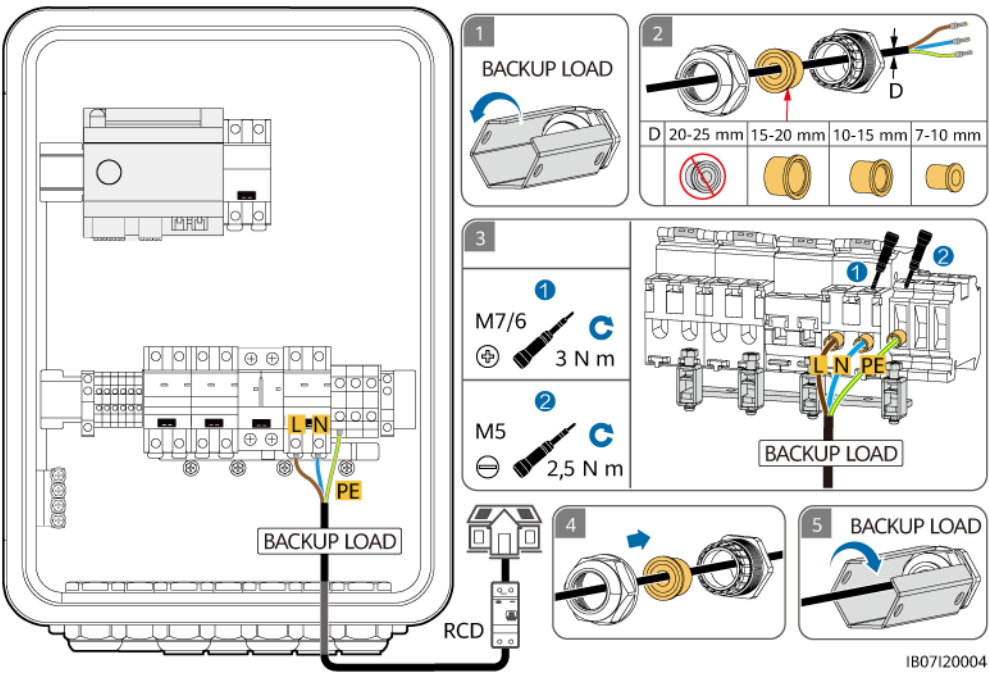
Figure 5-14 Connexion du câble d'alimentation de la charge de secours du SmartGuard-63A-S0
