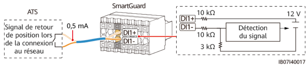
Figure D-1 Signal de retour de position lors de la connexion au réseau
