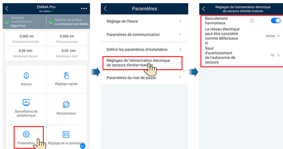
Figure 6-4 Réglages de l'alimentation électrique de secours d'entier-maison
