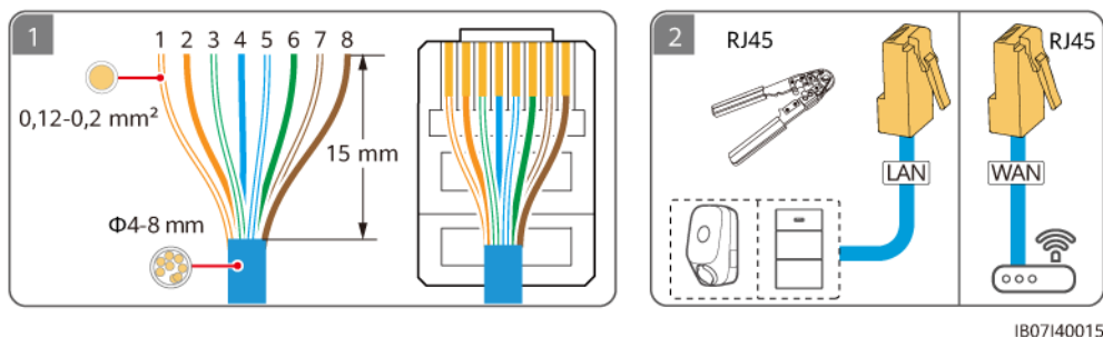
Figure 5-24 Câble de communication FE (les cases en pointillés indiquent les composants en option)
