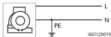
Figure 5-7 Mise à la terre des fils neutres du générateur
