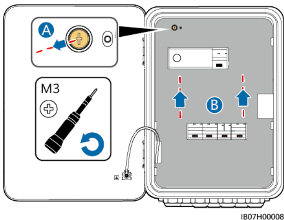
Figure 5-6 Ouverture du couvercle du compartiment de maintenance
