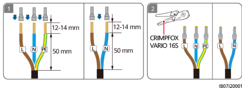
Figure 5-8 Sertissage des bornes d'extrémité du cordon CA
