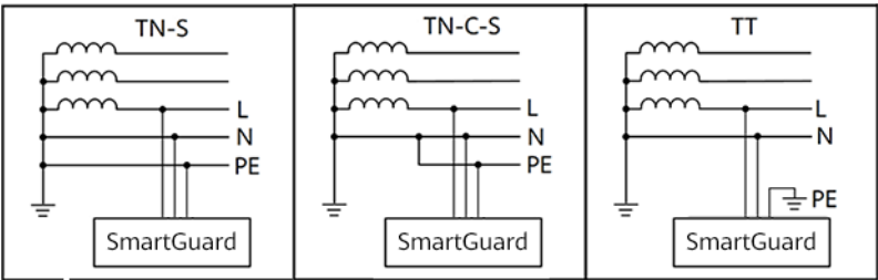
Figure 2-7 Systèmes de mise à la terre
