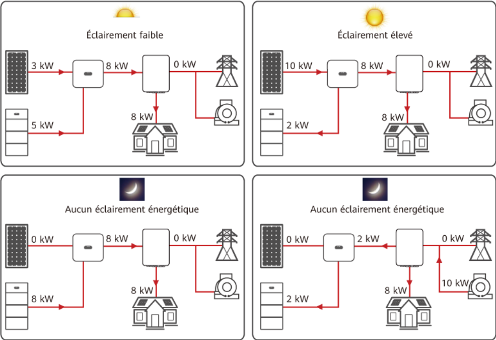
Figure 2-6 Illustration de la puissance maximale en mode hors réseau
