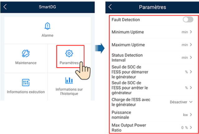
Figure 6-9 Configuration des paramètres du générateur
