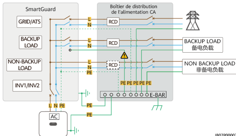
Figure 2-2 Schéma de câblage résidentiel du SmartGuard-63A-S0 (les lignes pointillées indiquent les connexions de câble optionnelles)
