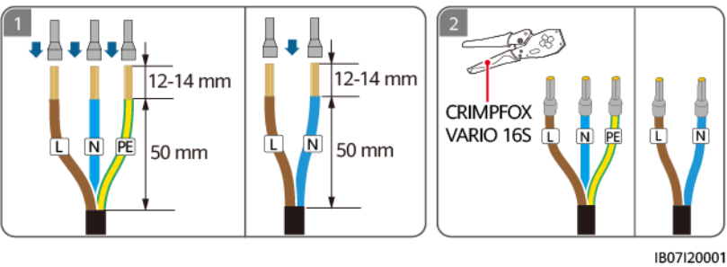
Figure 5-10 Sertissage des bornes d'extrémité du cordon CA
