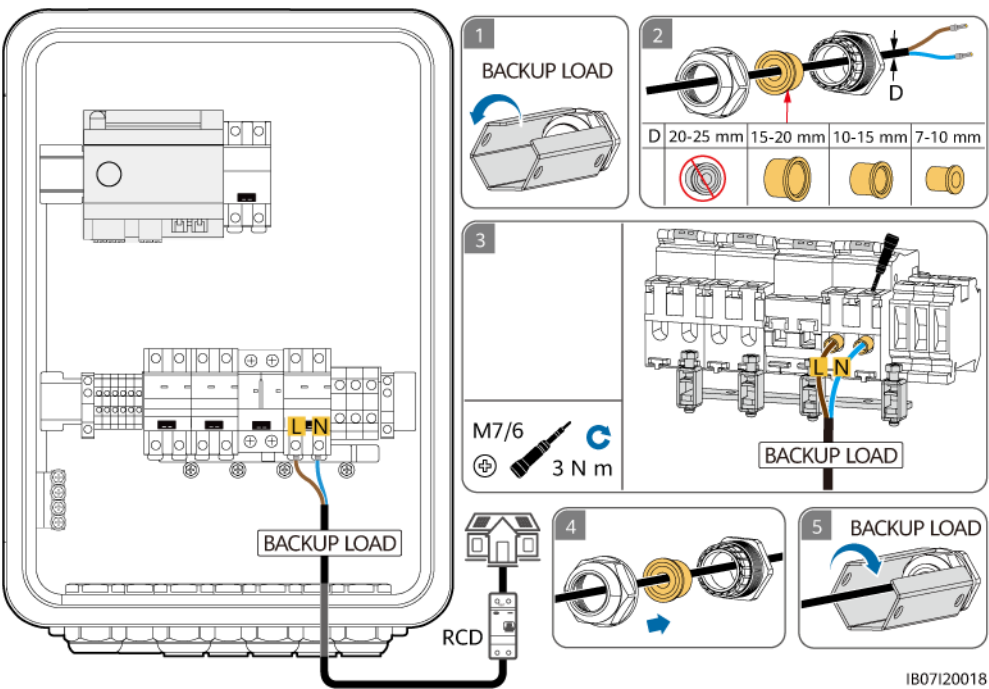
Figure 5-15 Connexion du câble d'alimentation de la charge de secours du SmartGuard-63A-AUS0
