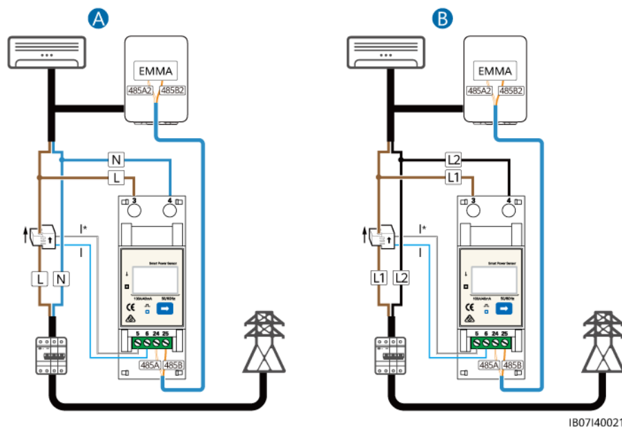
Figure 5-23 Connexion du câble de communication du compteur électrique
