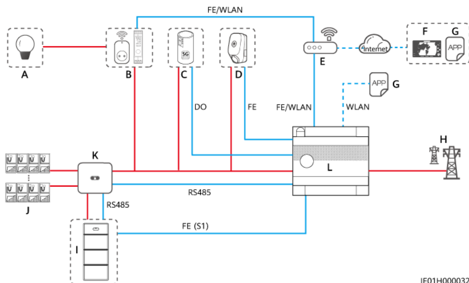
Figure 2-2 Diagramme de mise en réseau (en utilisant l'EMMA-A02 comme exemple)
