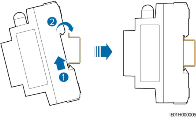
Figure 4-3 Installation de l'EMMA
