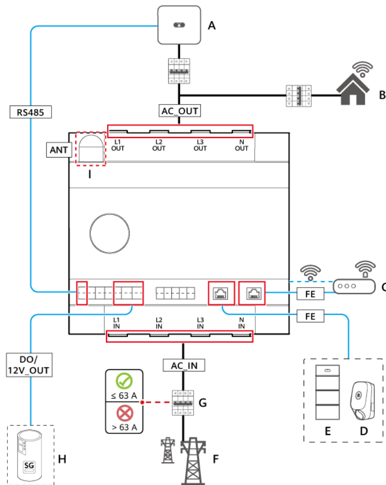
Figure 5-1 Diagramme de connexion des câbles : connexion CT interne (courant \leq 63 A)
