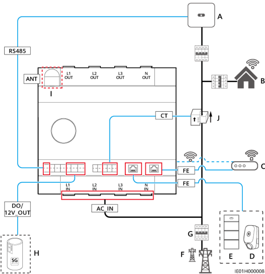
Figure 5-2 Diagramme de connexion des câbles : connexion CT externe (courant > 63 A)
