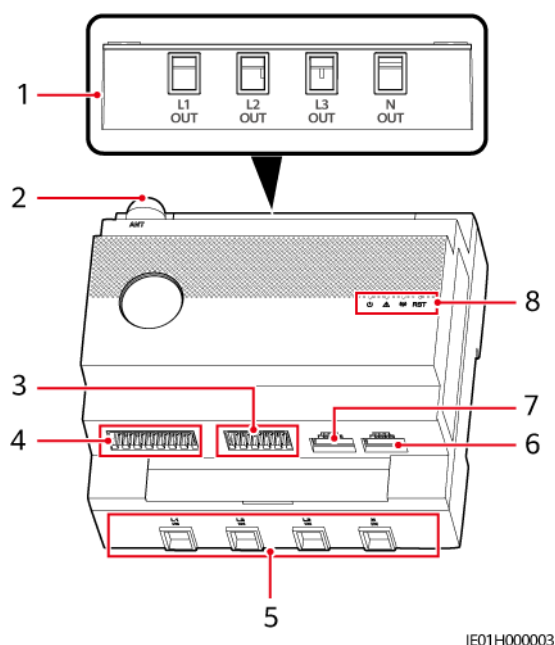
Figure 2-3 Description de l'aspect visuel
