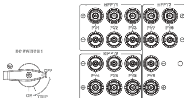
Figure 5-10 Terminaux CC contrôlés par DC SWITCH 1
