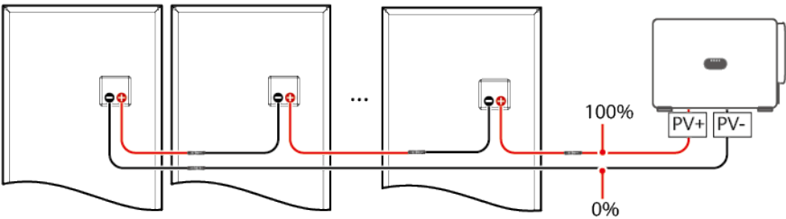
Figure 8-16 Définition du pourcentage de la localisation de court-circuit
