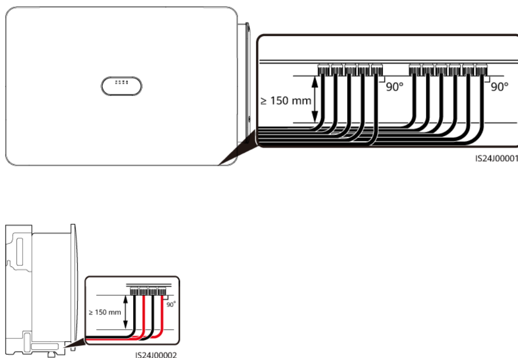
Figure 5-14 Exigences en matière de câblage d'alimentation d'entrée CC
