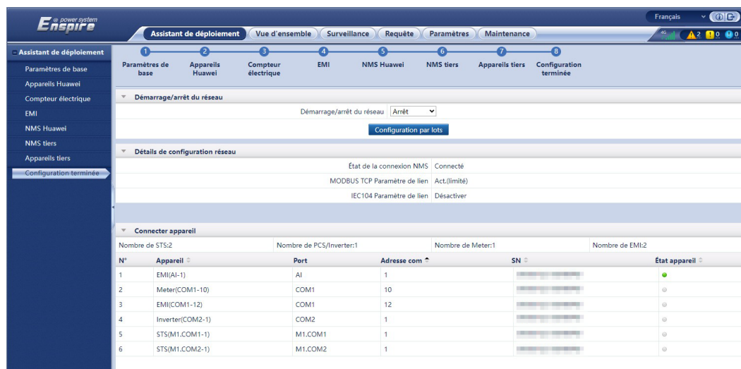
Figure 7-10 Fin de la configuration
