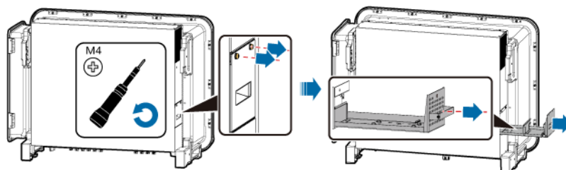
Figure 8-2 Retrait du plateau du ventilateur (1)
