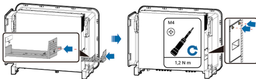
Figure 8-15 Réinstallation du plateau du ventilateur
