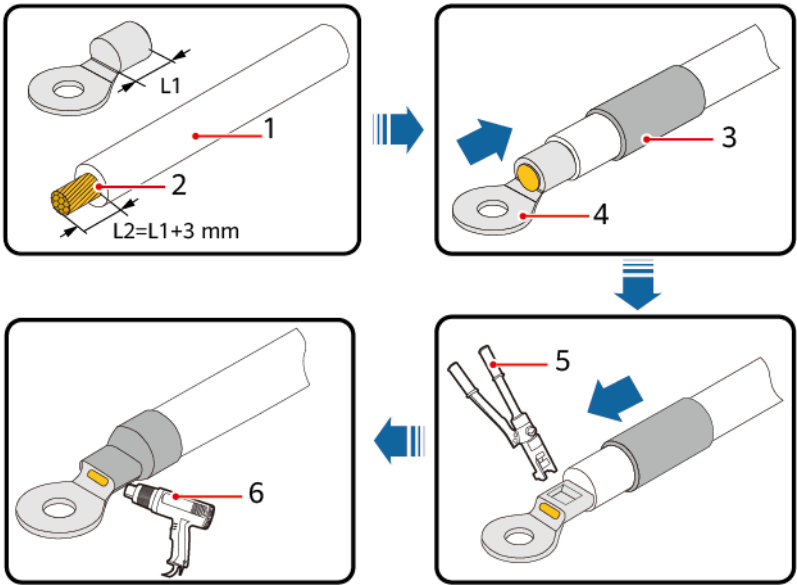
Figure D-2 Sertissage d'une borne OT
