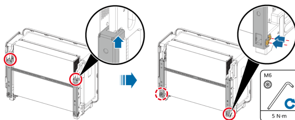
Figure 4-16 Fixation de l'onduleur
