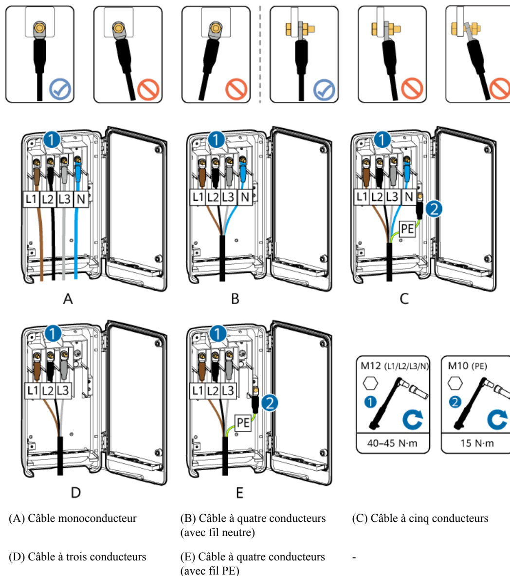
Figure 5-6 Connexion des câbles
