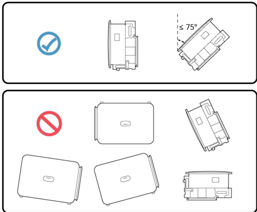
Figure 4-7 Angle d'installation
