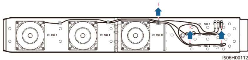
Figure 8-7 Retrait des attaches de câbles du FAN 3
