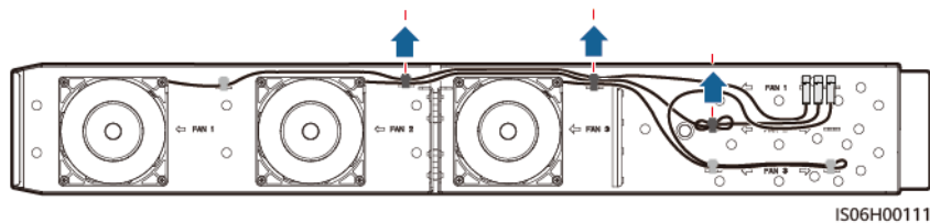
Figure 8-6 Retrait des attaches de câbles du FAN 2
