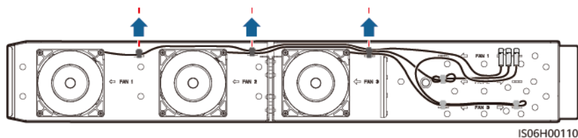
Figure 8-5 Retrait des attaches de câbles du FAN 1
