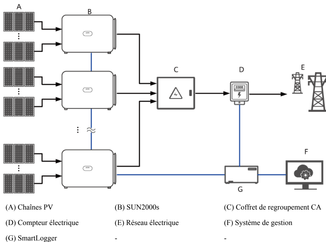
Figure 2-2 Application de mise en réseau RS485 (SmartLogger)
