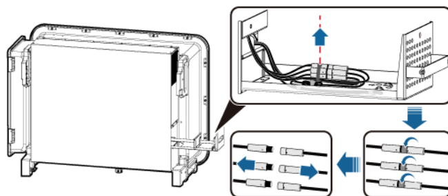
Figure 8-3 Déconnexion des câbles
