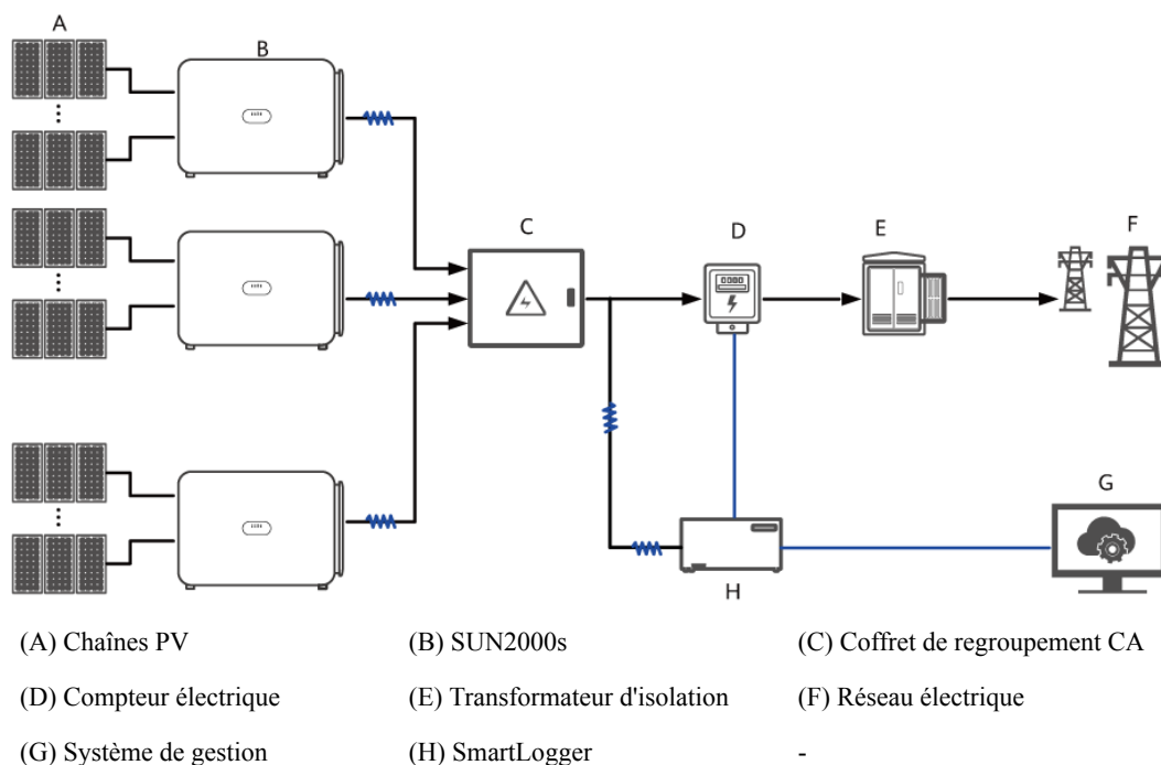
Figure 2-4 Application de mise en réseau du MBUS (SmartLogger)
