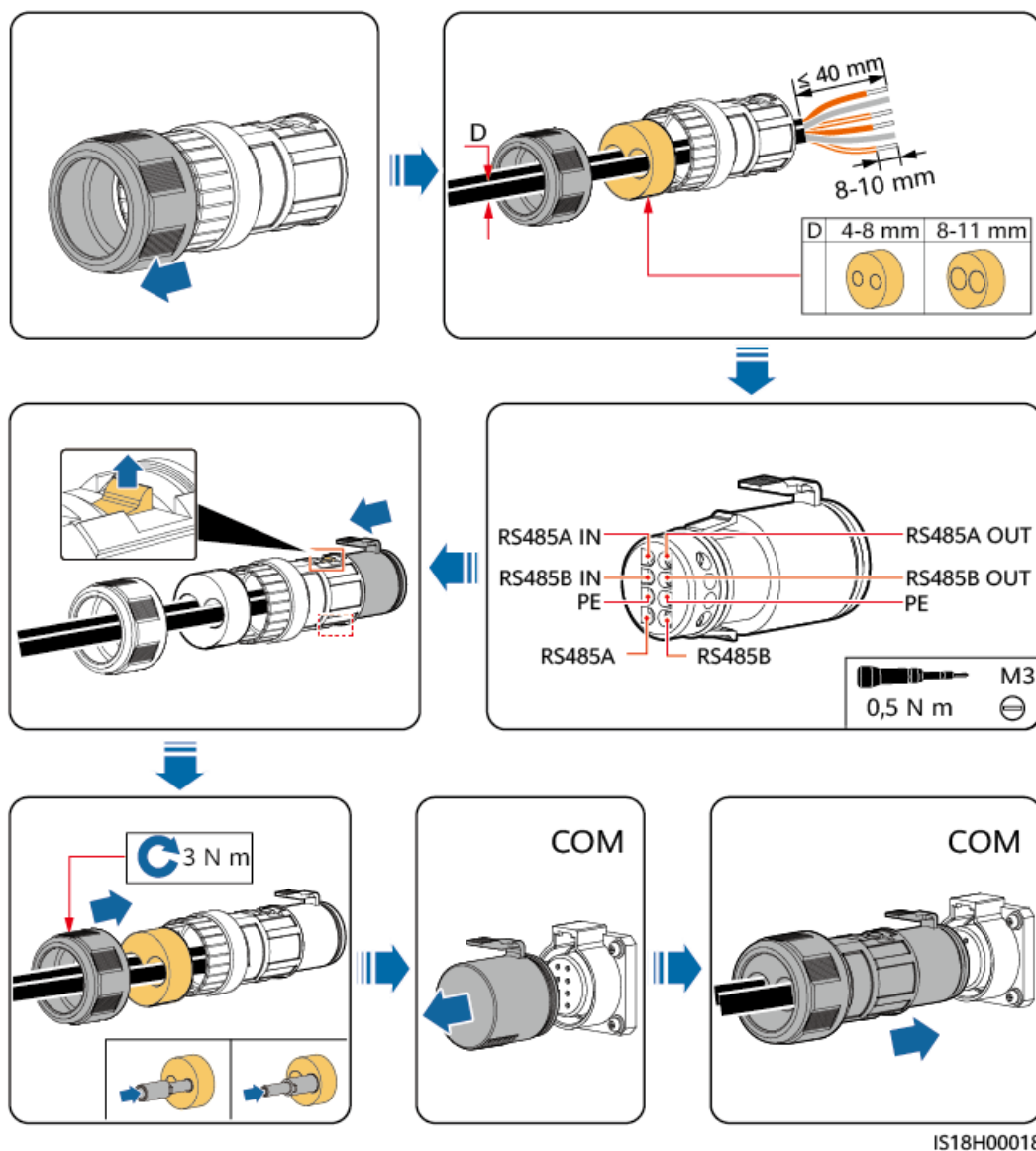
Figure 5-19 Connexion des câbles de communication
