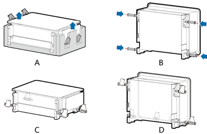
Figure 4-8 Déballage, déplacement et montage de l'onduleur
