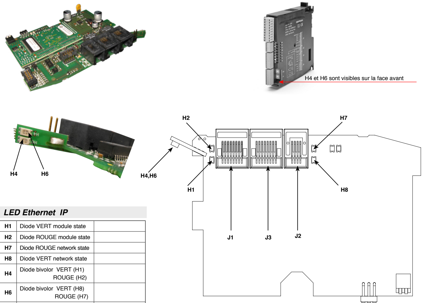
Figure 28 Port2: Interface Modbus RTU / Ethernet IP ou Modbus RTU/EtherCAT ou Modbus RTU / ProfiNET
