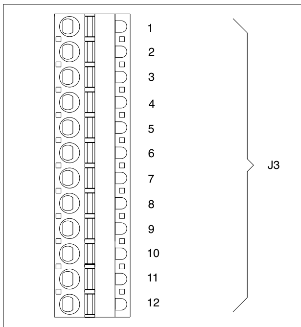
Figure 16 Schéma de raccordement des sorties 1...4 du type logique
