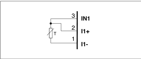
Figure 19 Schéma de raccordement de l'entrée du type Pt100
