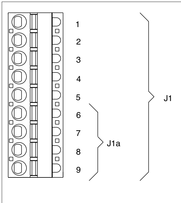
Figure 8 Connecteur J1
