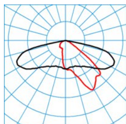
Jovie 50-AB2L-2-10-740-CLO-E DIN 5040 2 = A30 CEN flux code = 35 71 96 100 100 UGR I 2 = 0,0 UGR q 2 = 0,0 UTE 2 = 1.00 G
