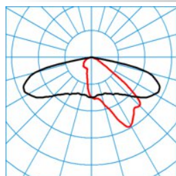
Jovie 50-AB2L-2-10-740-CLO-B DIN 5040 = A30 CEN flux code = 35 71 96 100 100 UGR I = 0,0 UGR q = 0,0 UTE = 1.00 G
