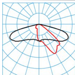
Jovie 50-AB2L-4-32-740-CLO-B DIN 5040 = A30 CEN flux code = 35 72 98 100 100 UGR I = 0,0 UGR q = 0,0 UTE = 1.00 G
