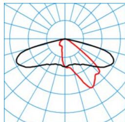
Jovie 50-AB2L-4-32-740-CLO-E DIN 5040 2 = A30 CEN flux code = 35 72 98 100 100 UGR I 2 = 0,0 UGR q 2 = 0,0 UTE 2 = 1.00 G
