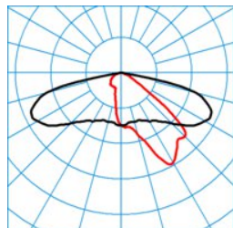
Jovie 50-AB2L-2-22-730-CLO-E DIN 5040 2 = A30 CEN flux code = 35 71 96 100 100 UGR I 2 = 0,0 UGR q 2 = 0,0 UTE 2 = 1.00 G
