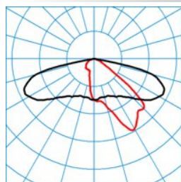
Jovie 50-AB2L-2-22-730-CLO-B DIN 5040 = A30 CEN flux code = 35 71 96 100 100 UGR I = 0,0 UGR q = 0,0 UTE = 1.00 G
