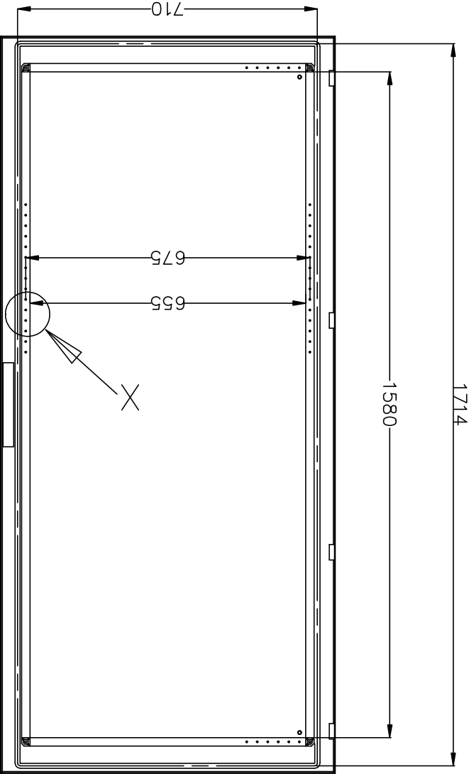
VISTA POSTERIOR PUERTA DOOR REAR VIEW
