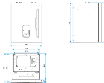
Unité supérieure T.One® AquaAIR avec façade
