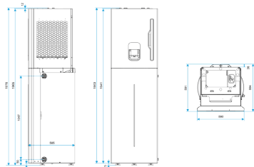
Unité intérieure T.One® AquaAIR version premium
