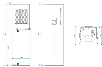
Unité intérieure T.One® AquaAIR version premium
